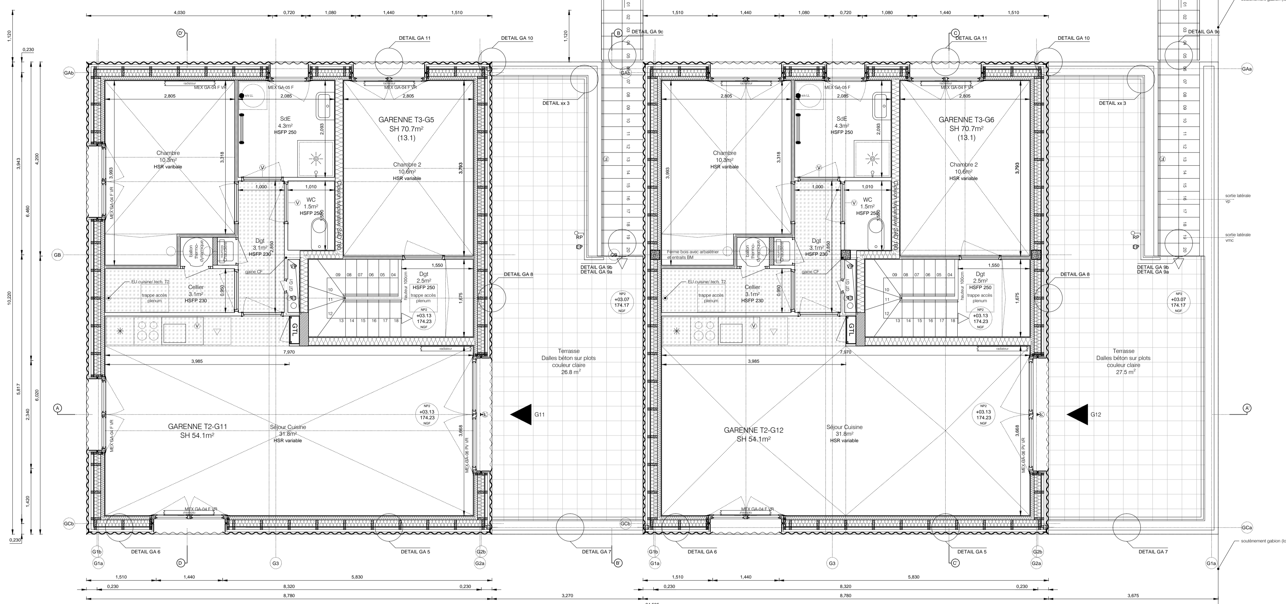
GARENNE G5 G6 (T3) + G11 G12 (T2) PLAN R+1 - échelle 1/50e
