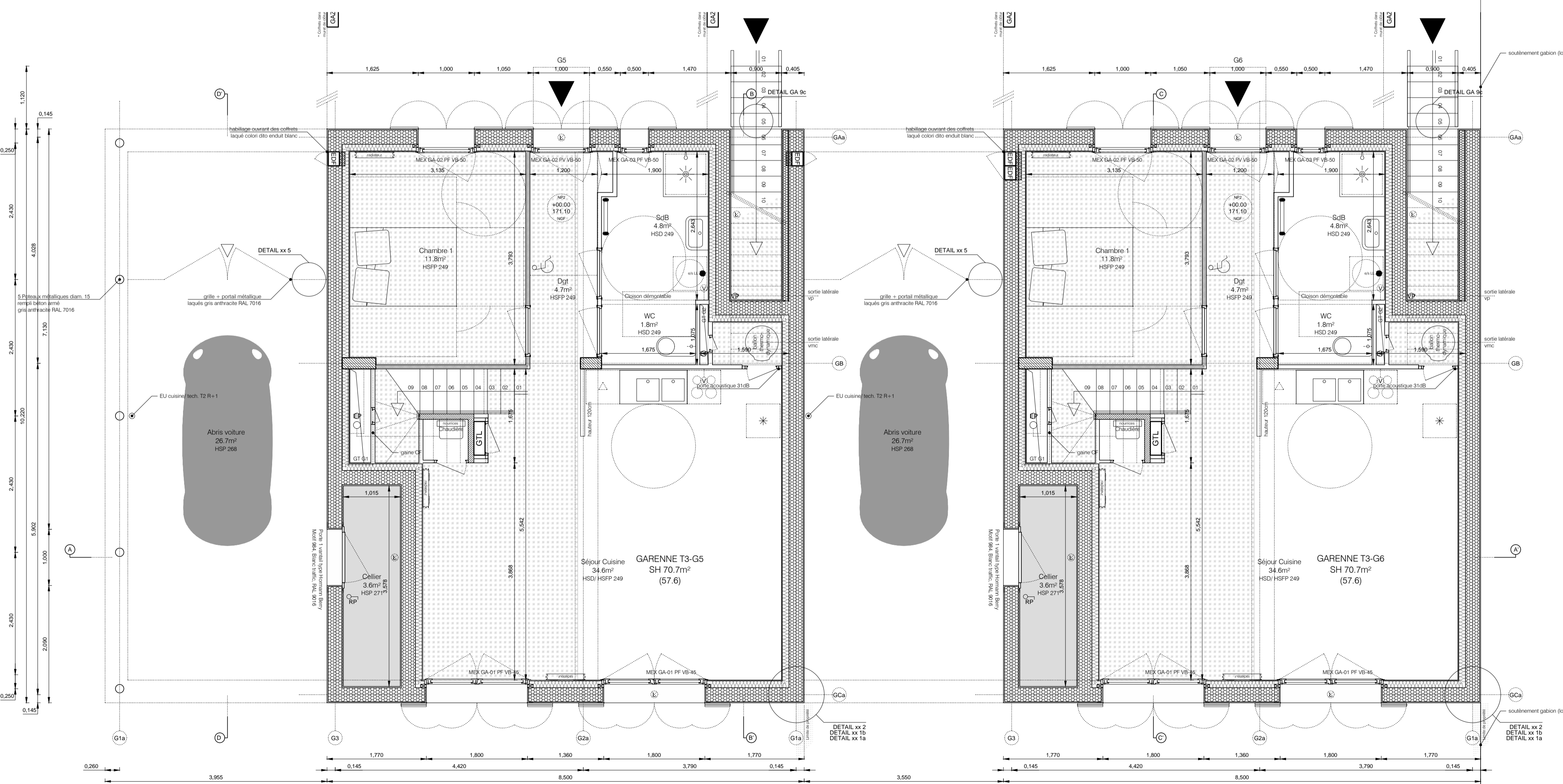
GARENNE G5 G6 (T3) + G11 G12 (T2) PLAN DE Rdc - échelle 1/50e
