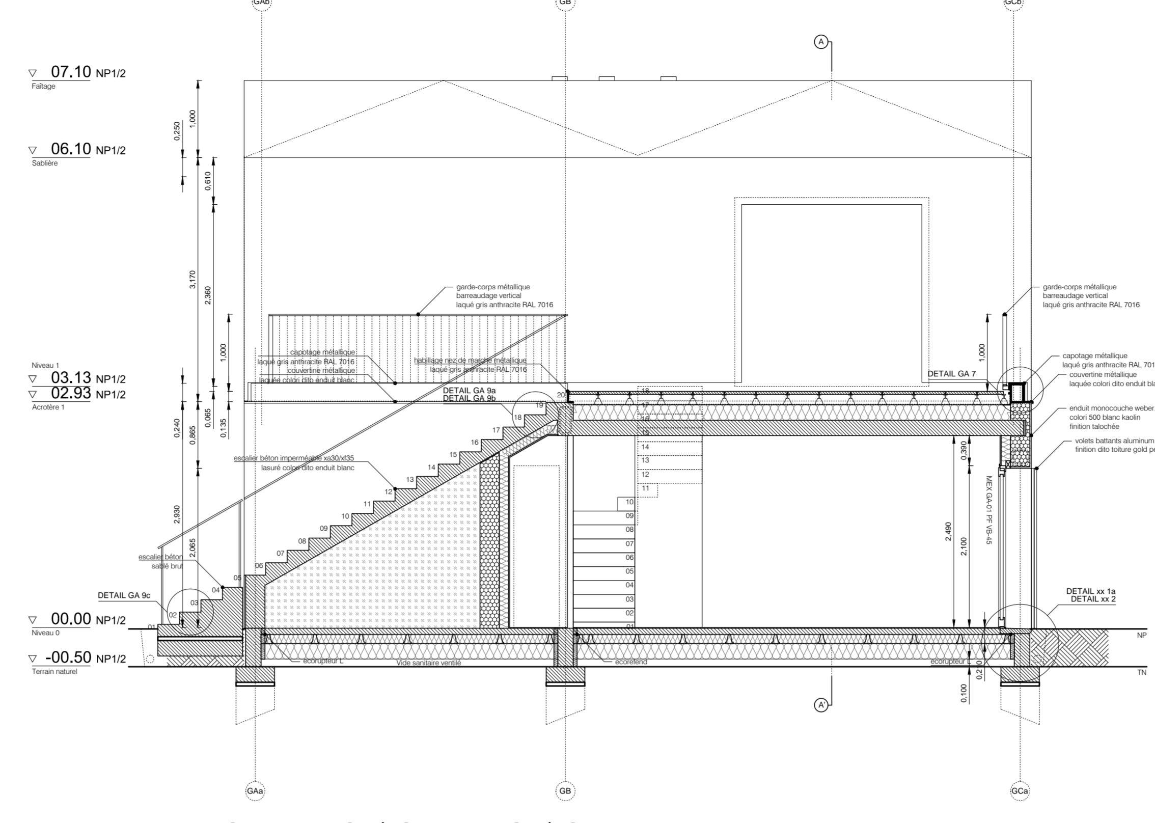
GARENNE G1 à G6 (T3) + G7 à G12 (T2) COUPE BB' transversale - échelle 1/50e
