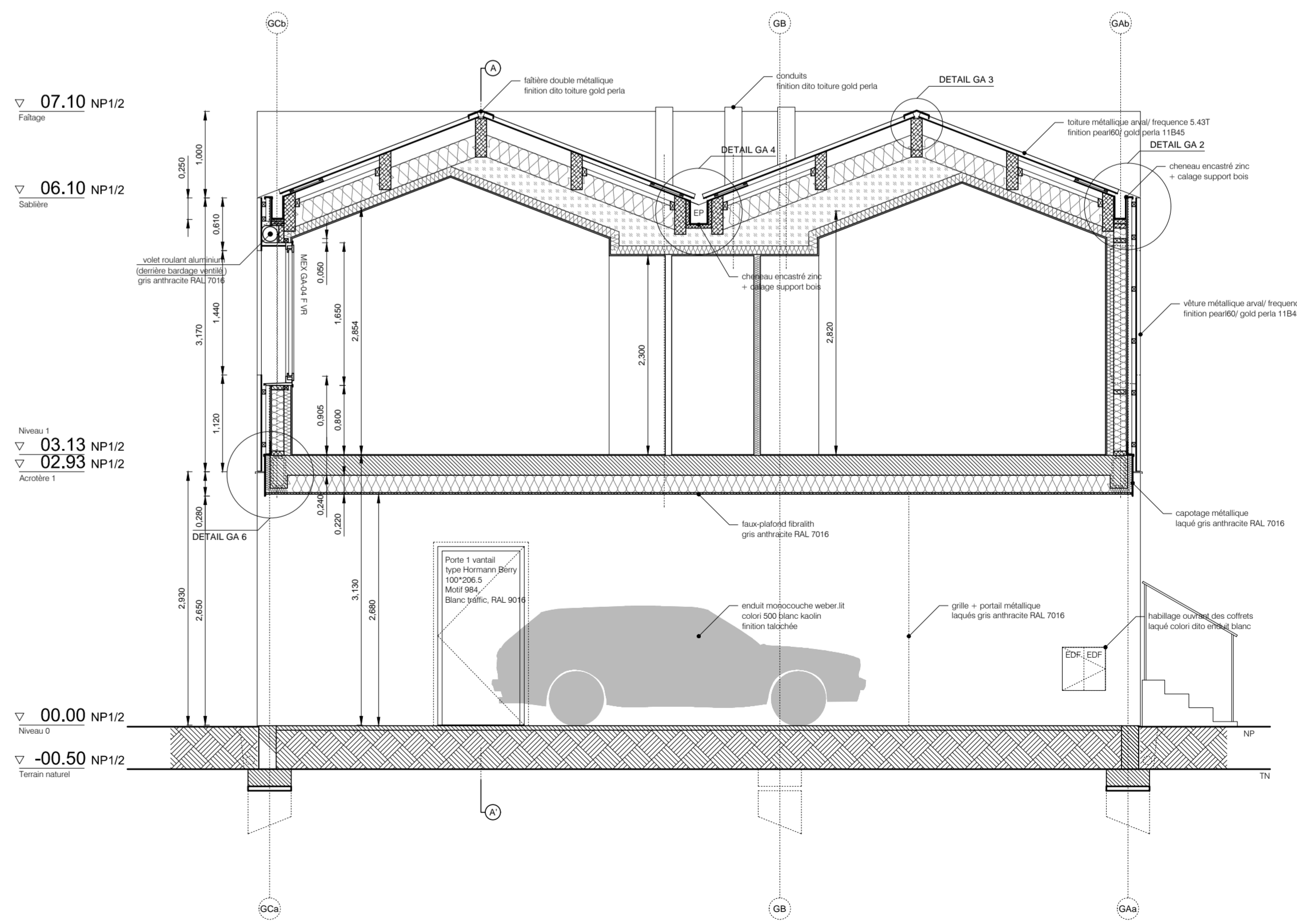
GARENNE G1 à G6 (T3) + G7 à G12 (T2) COUPE DD' transversale - échelle 1/50e
