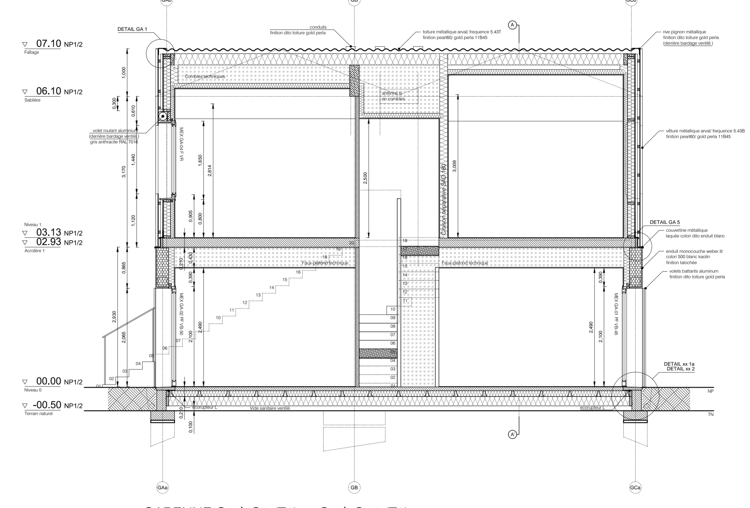
GARENNE G1 à G6 (T3) + G7 à G12 (T2) COUPE CC' transversale - échelle 1/50e
