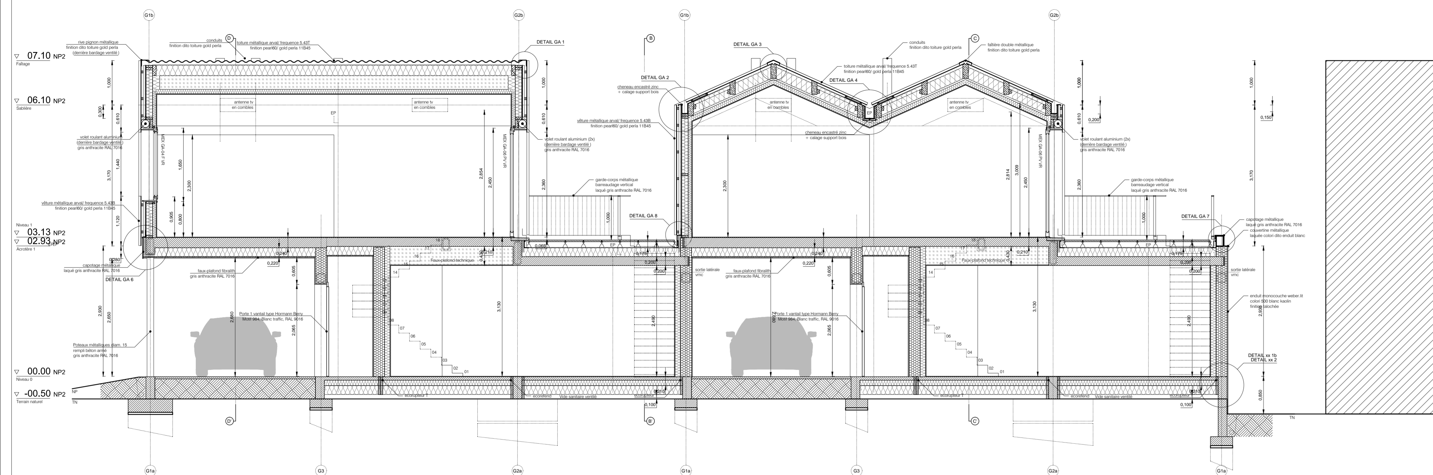
GARENNE G5 G6 (T3) + G11 G12 (T2) COUPE AA' longitudinale - échelle 1/50e
