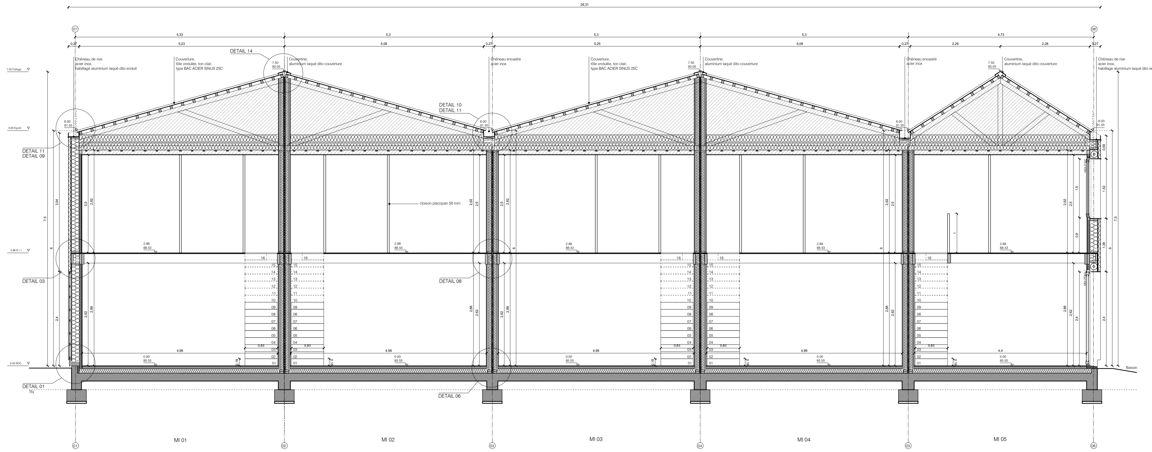
COUPE TRANSVERSALE /// MI01 à MI05
