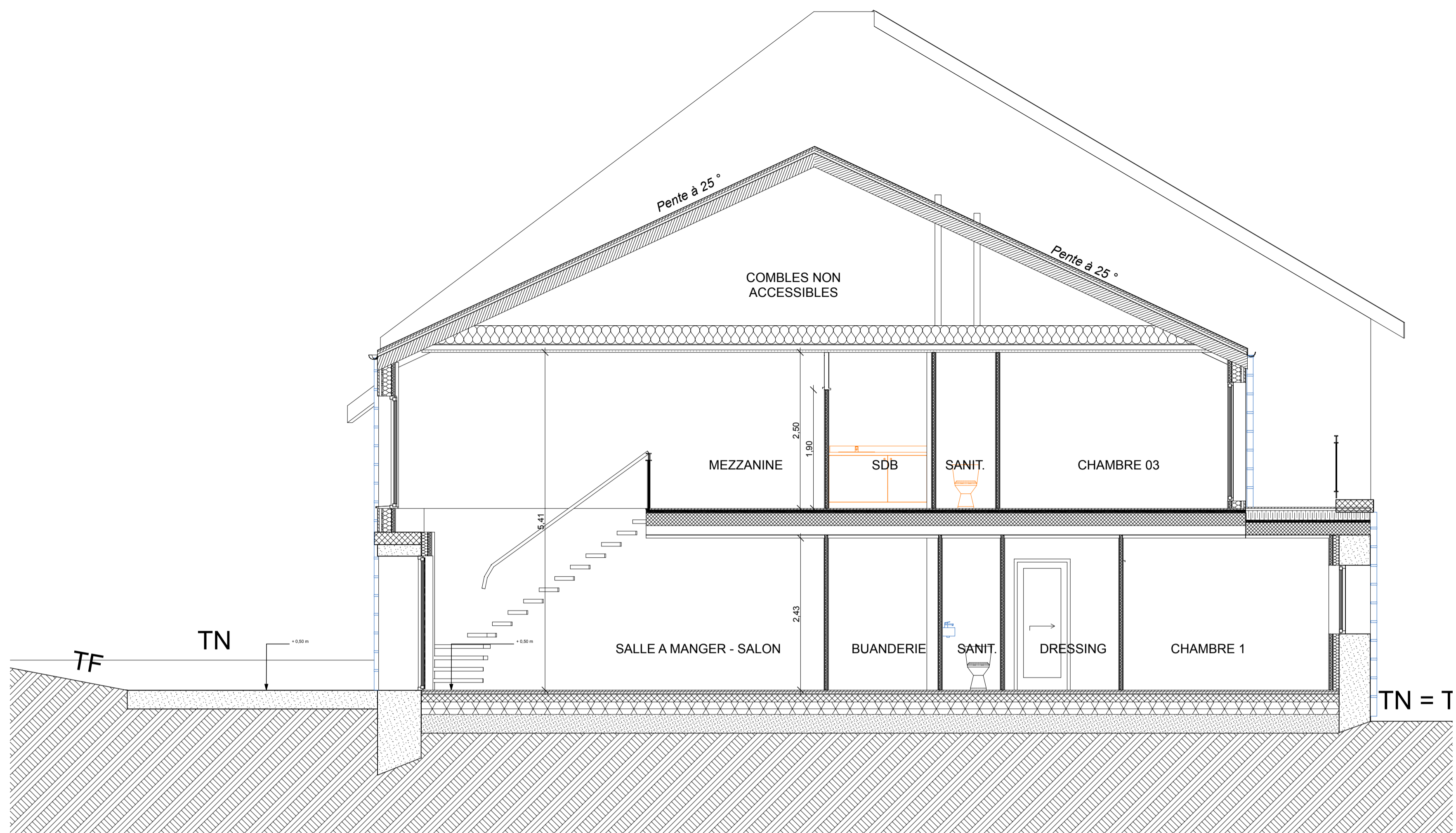
Coupe BB
