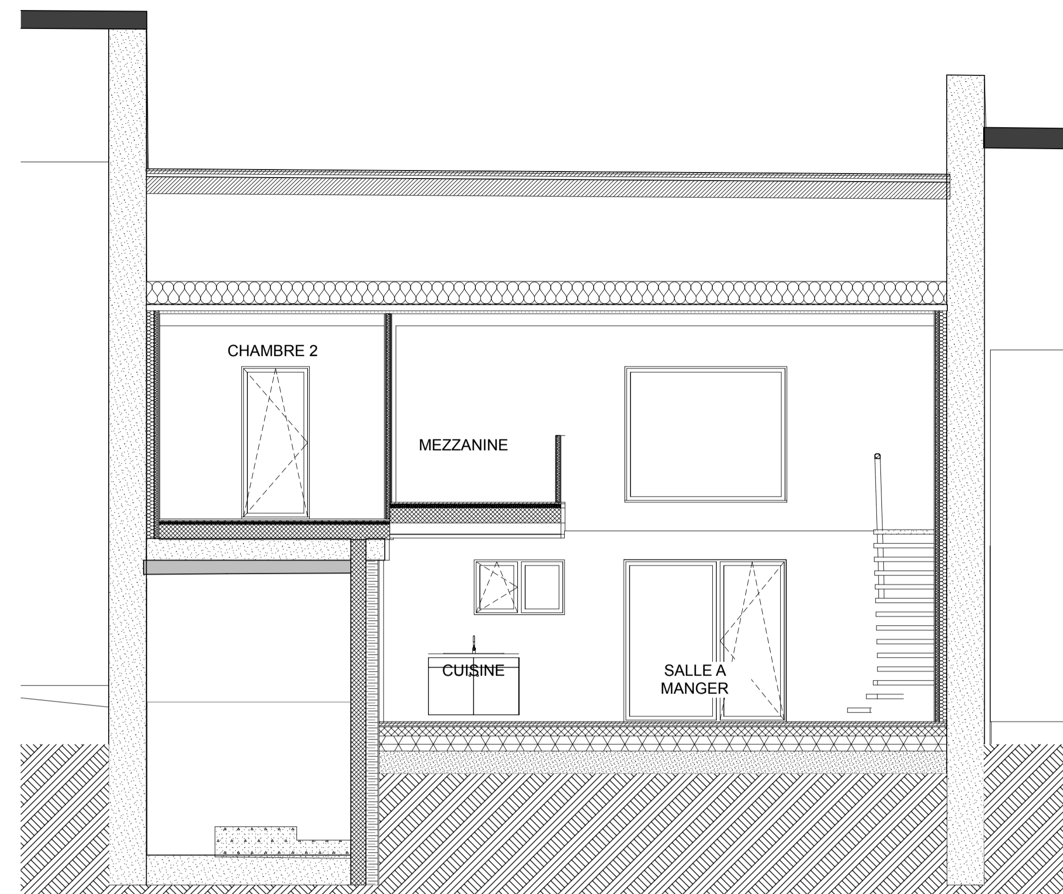
Coupe AA
