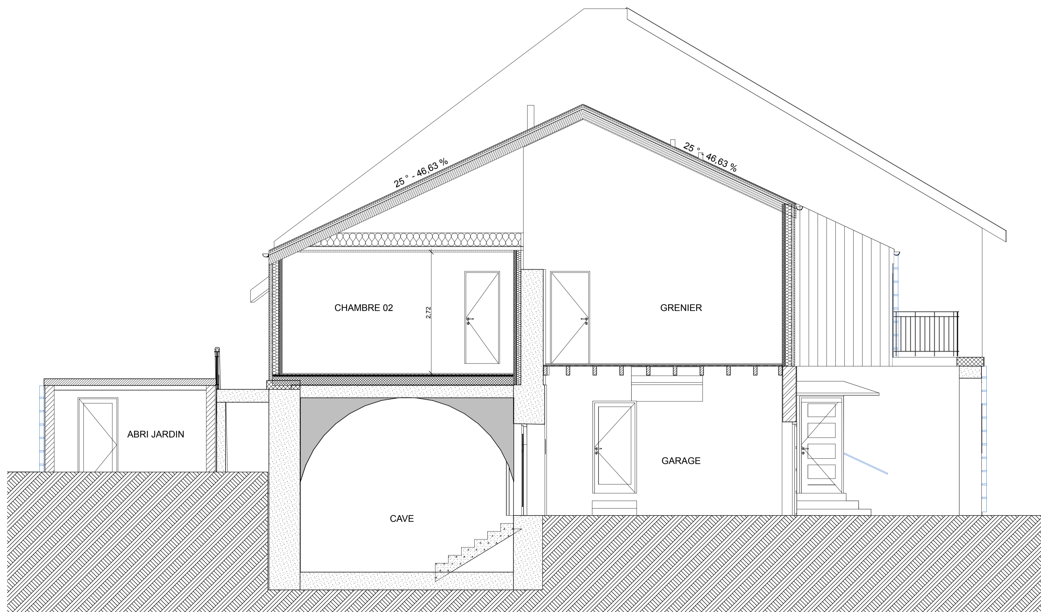
Coupe BB
