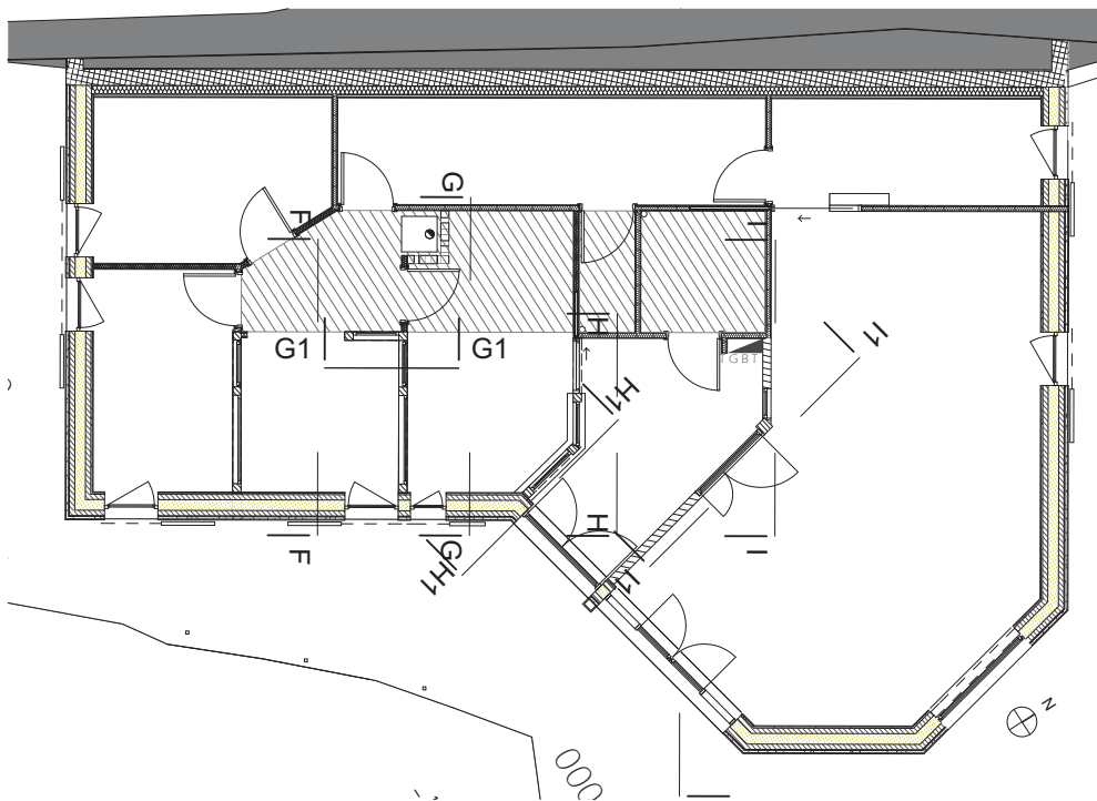
Dimensions similaires pour coupe FF G Coupe GG 1:50 Fen-005 Fen-003 Fen-007 Briques terre compressée en moucharabieh G1 Coupe GG 1:50
