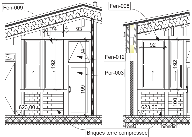
H Coupe HH 1:50 H1 Coupe HH 1:50 Fen-009 Fen-008 Fen-012 Por-003 Briques terre compressée
