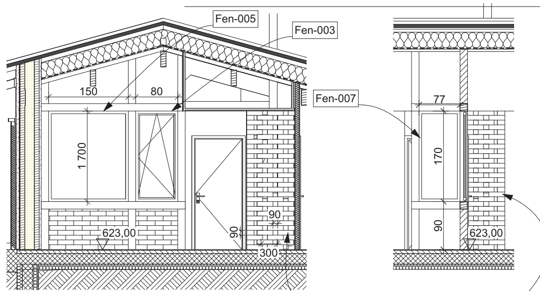
Dimensions similaires pour coupe FF G Coupe GG 1:50 Fen-005 Fen-003 Fen-007 Briques terre compressée en moucharabieh G1 Coupe GG 1:50
