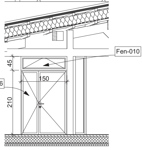
I1 Coupe II 1:50 Fen-010 Por-006
