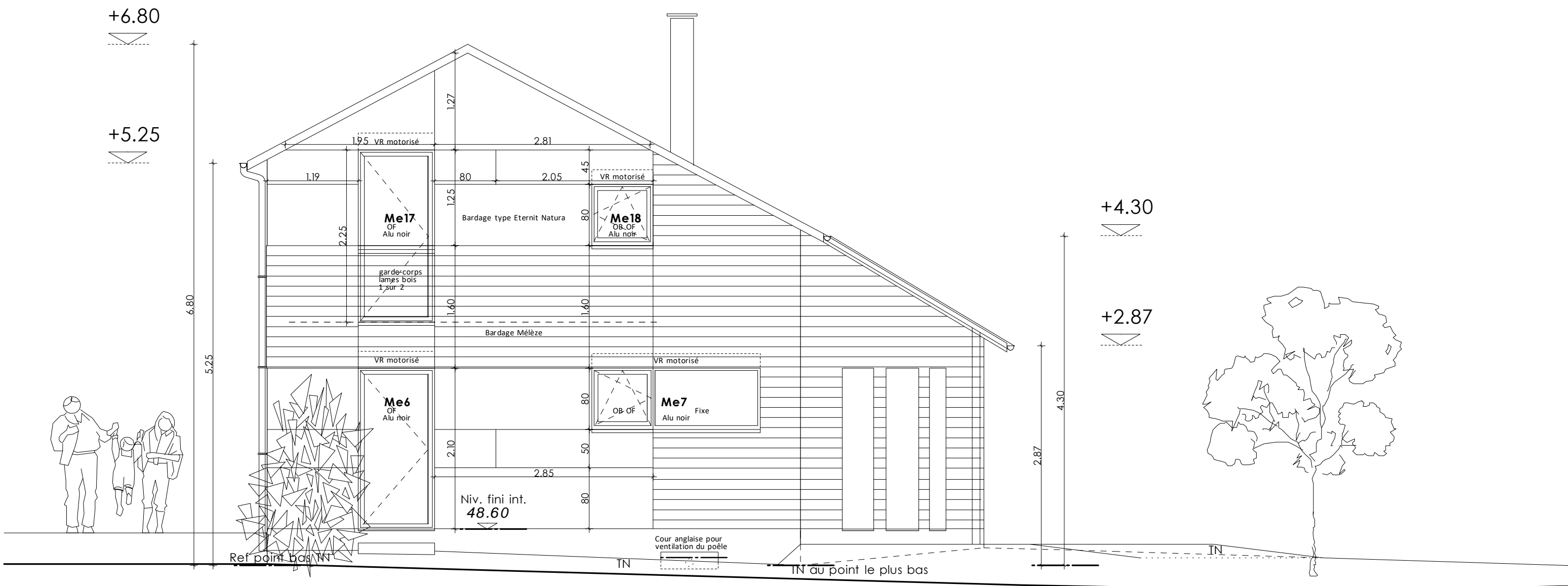
Façade Nord Ouest
