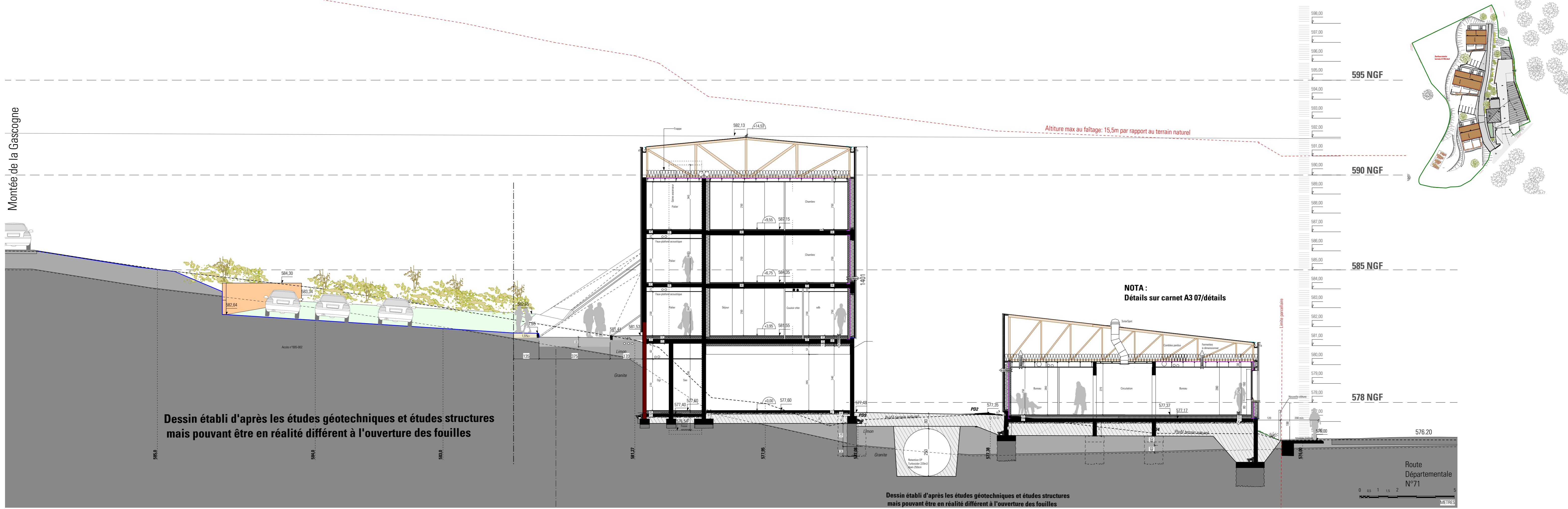
Coupe BB - Sur les bâtiment 001 et 006 (1/100ème)
