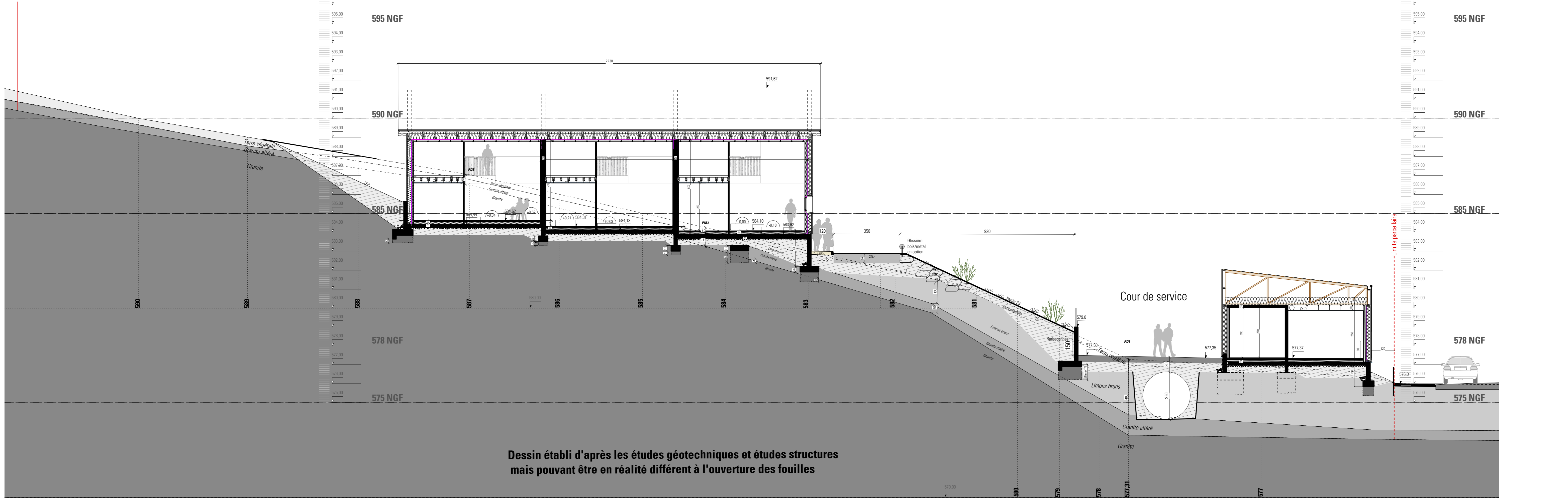
Coupe CCbis - Façade Sud bât 004 (1/100ème)
