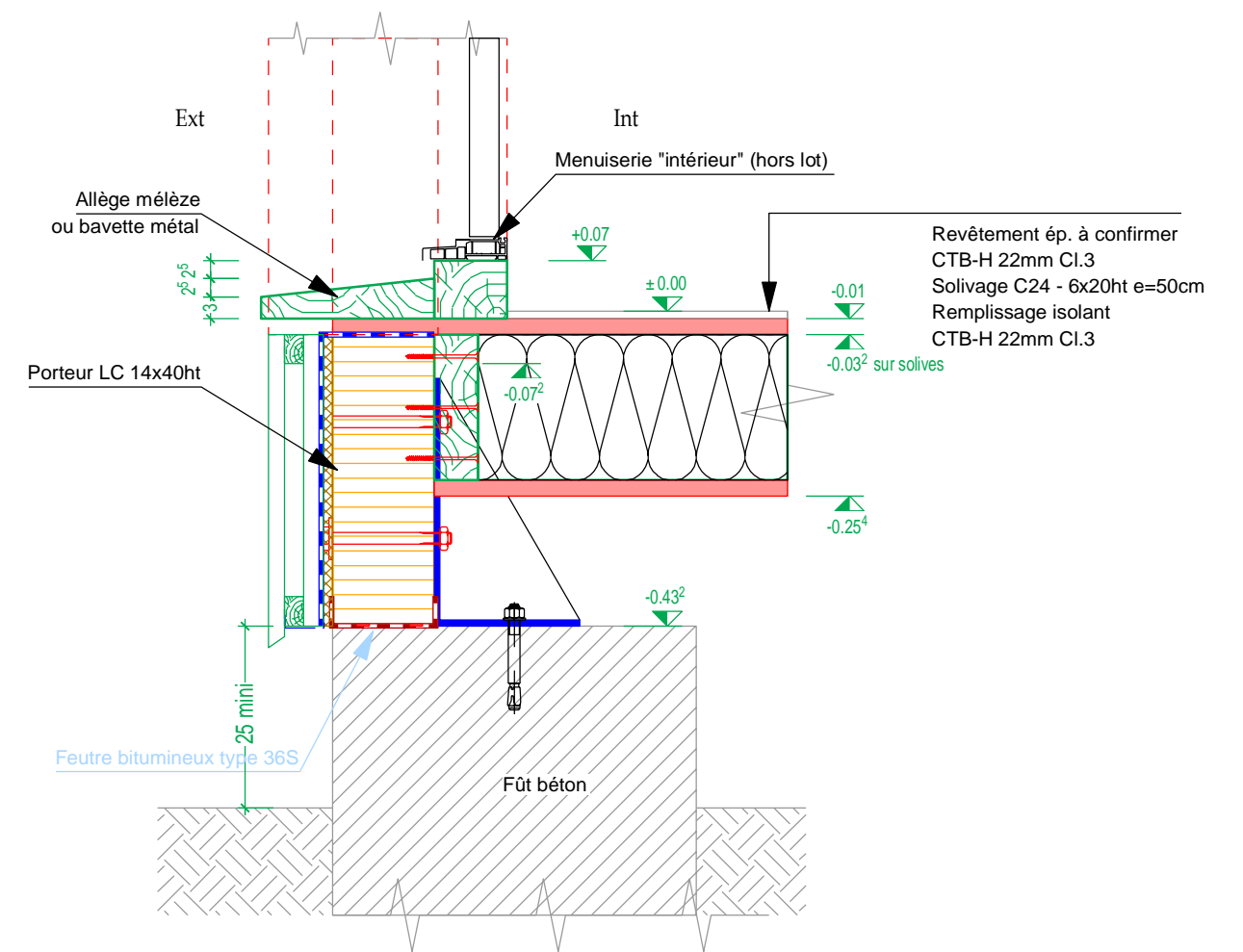
COUPE TYPE SEUIL SUR EXTERIEUR - Ech 1/10e
