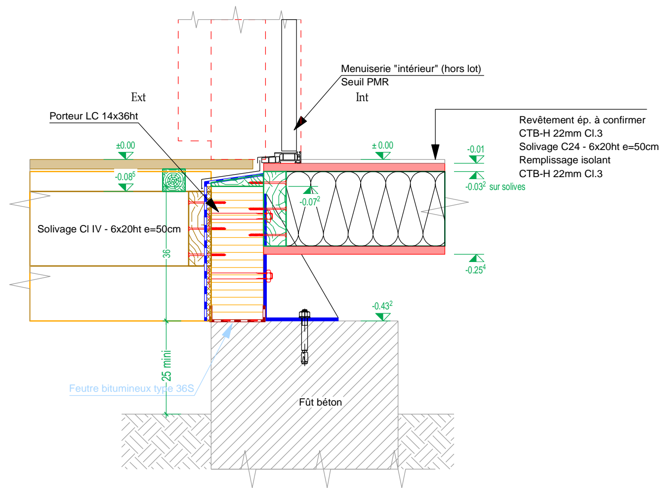
COUPE TYPE SEUIL TERRASSE ACCESSIBLE - Ech 1/10e
