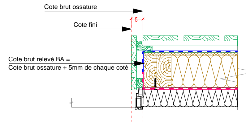
COUPE HORIZONTAL SUR MENUISERIE PATIO
