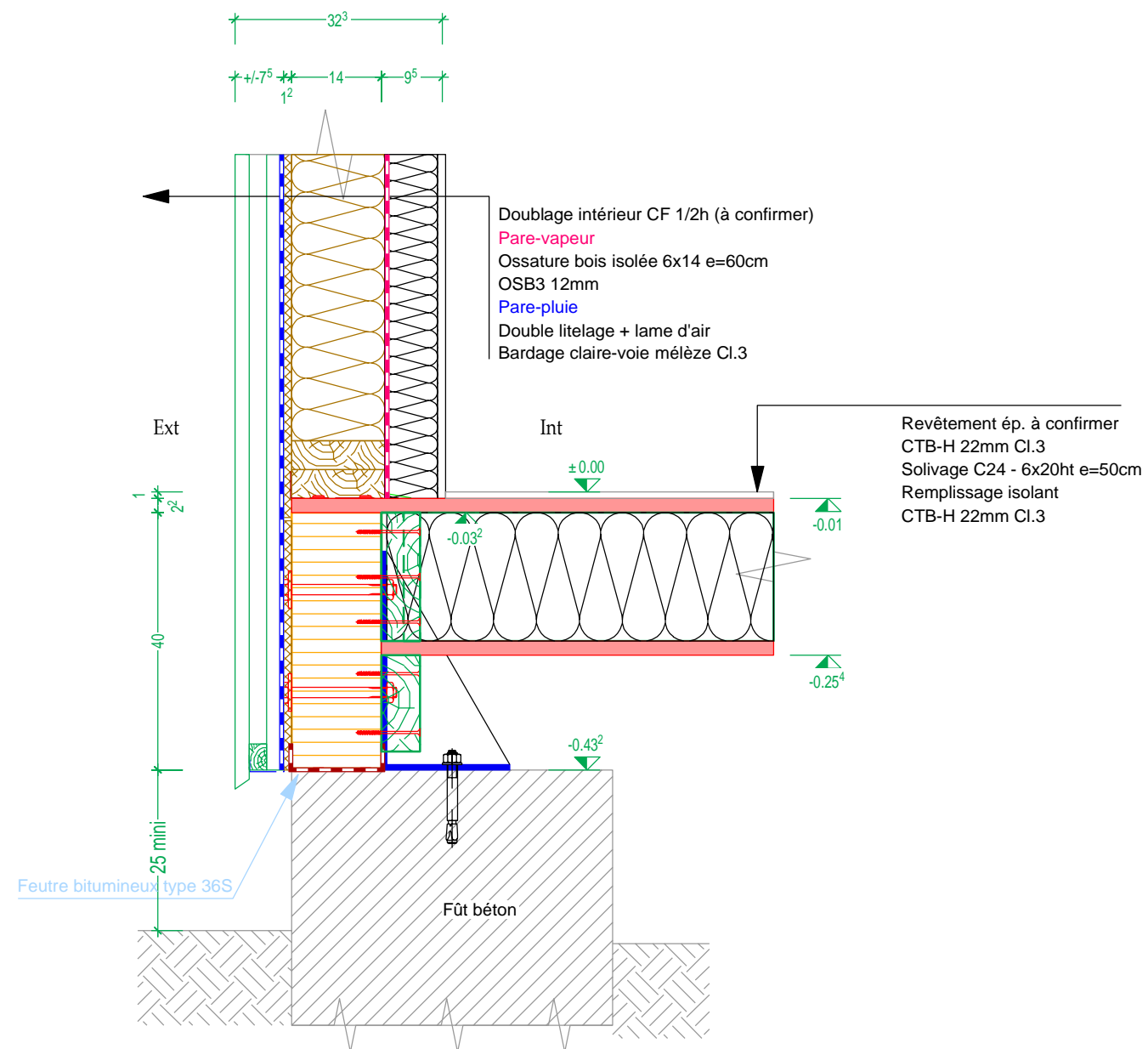
COUPE TYPE SUR PIED DE MUR EXTERIEUR - Ech 1/10e
