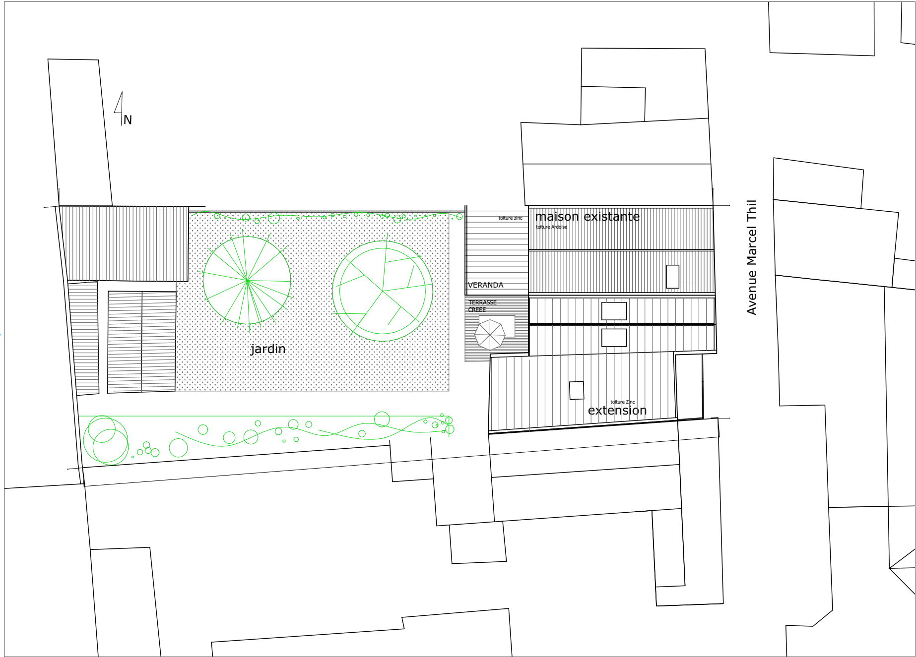
PLAN Masse - 1/200
