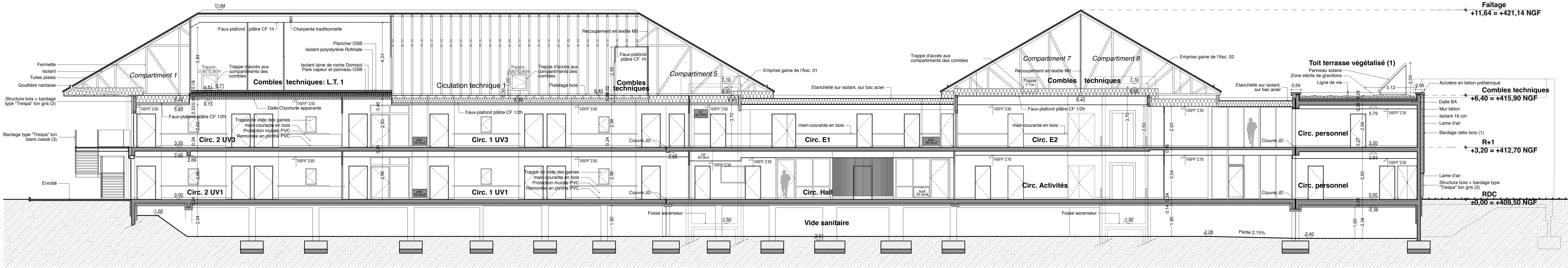
Coupe GG
