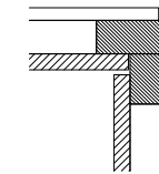
COUPE VERTICALE SUR PARTIE PORTE
