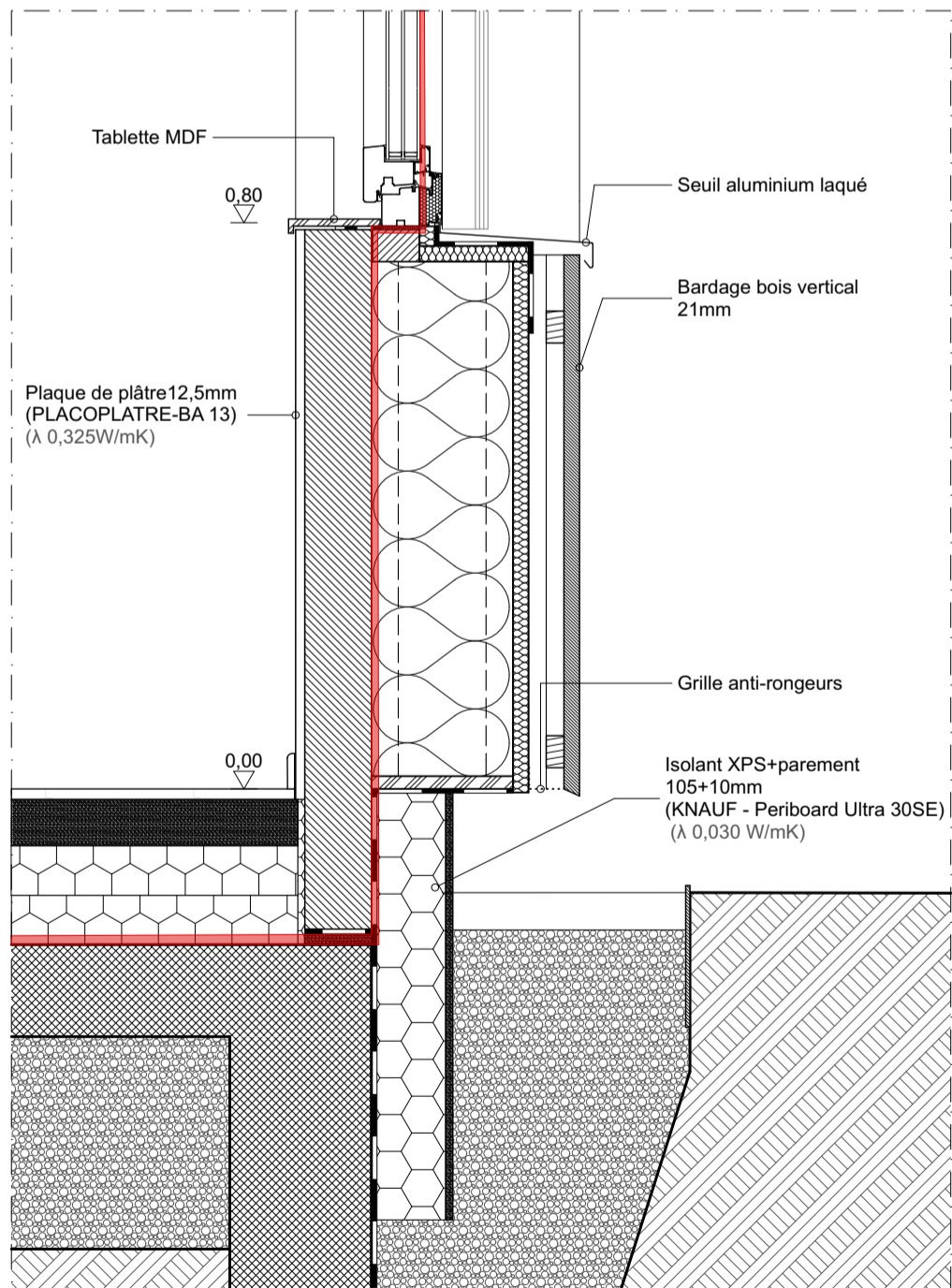
D-1.3 Détail fenêtre Sud: coupe verticale (inf.) 1:10
