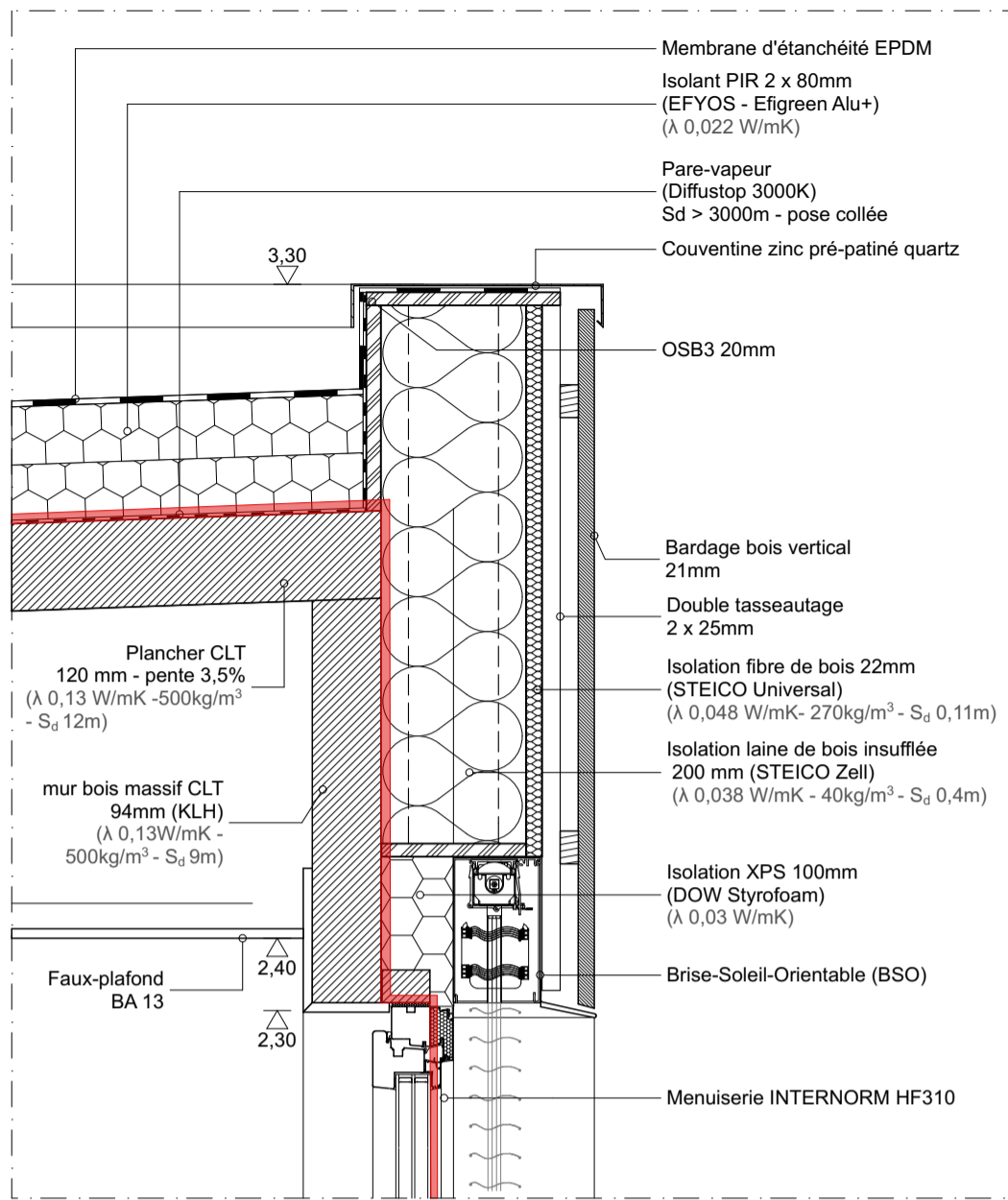
D-1.2 Détail fenêtre Sud: coupe verticale (sup.) 1:10
