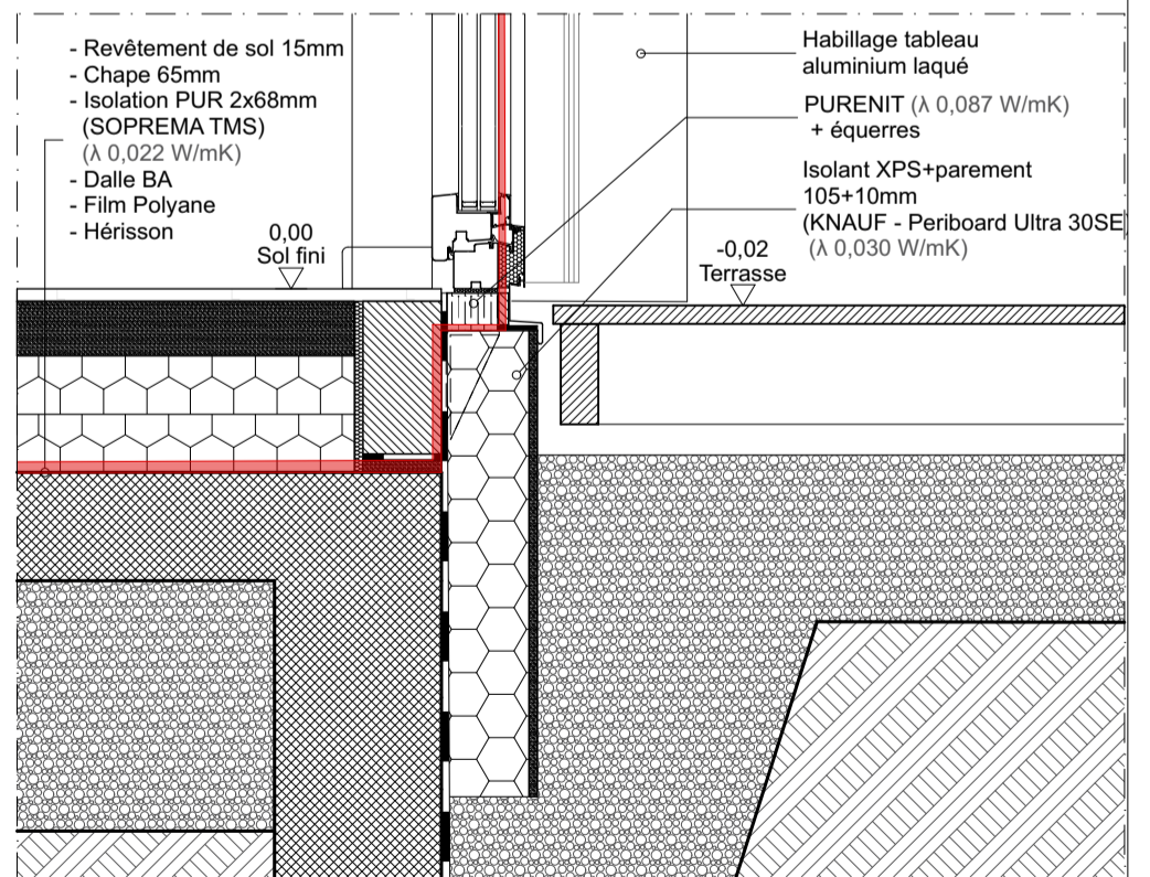
D-1.4 Détail porte fenêtre Sud: coupe verticale (inf.) 1:10
