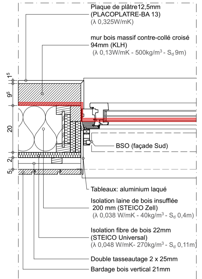
D-1.1 Détail fenêtre Sud: coupe horizontale 1:10
