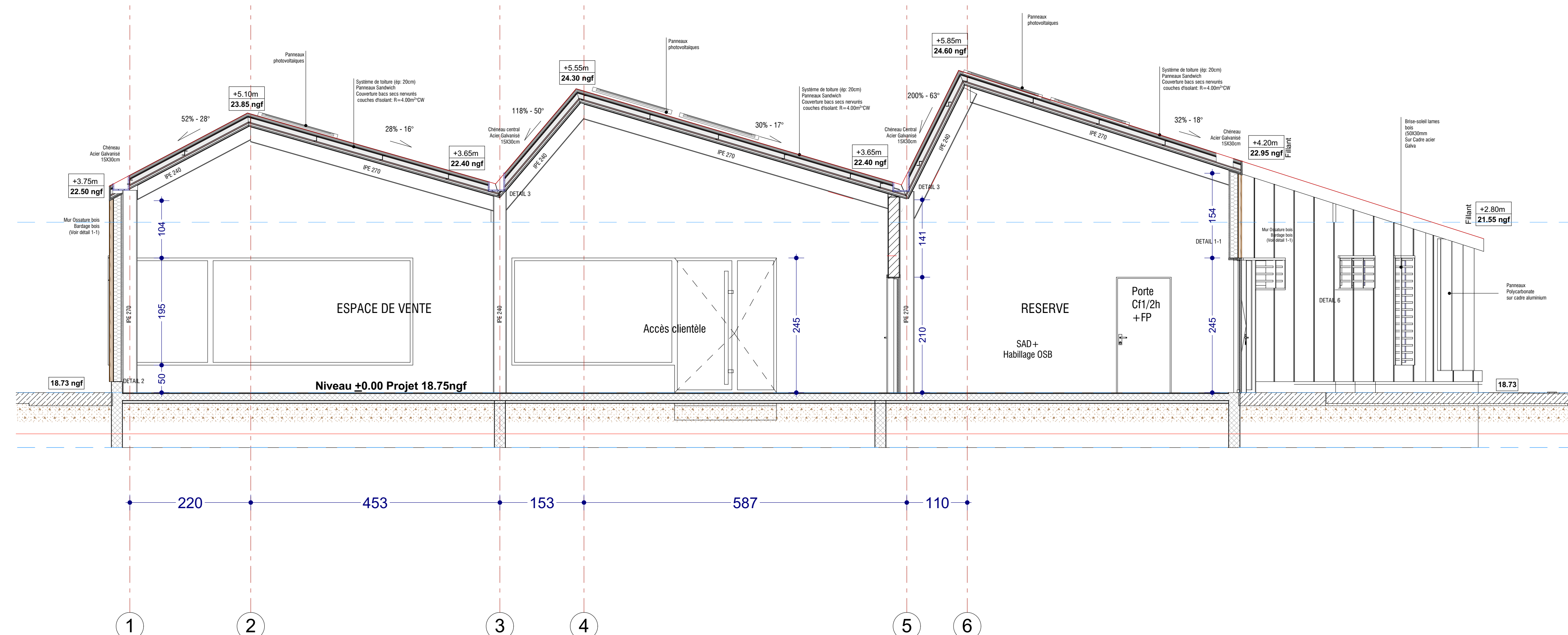
Coupe AA
