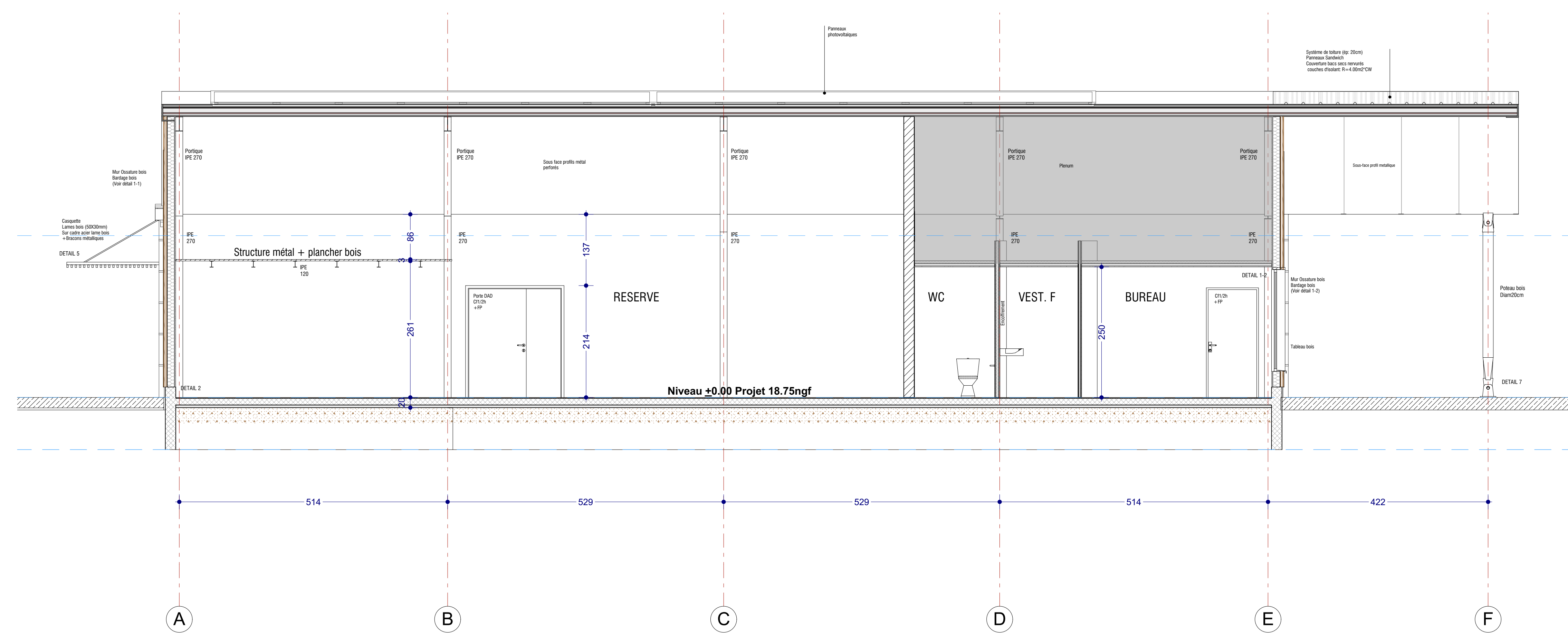
Coupe BB
