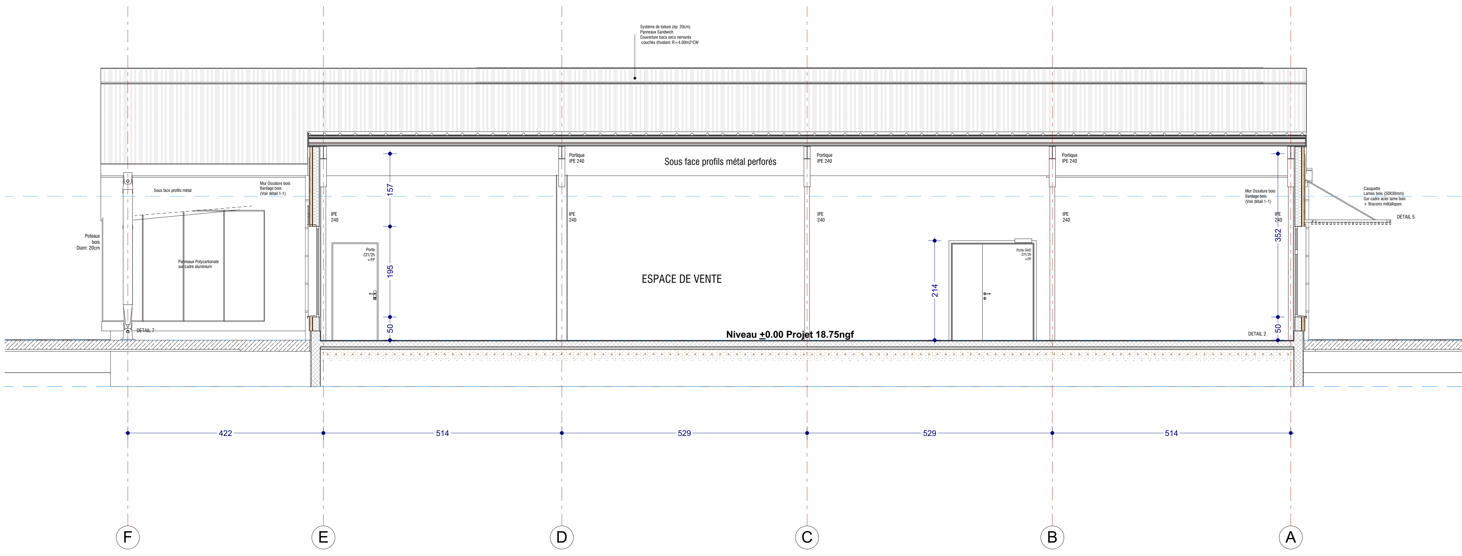
Coupe CC
