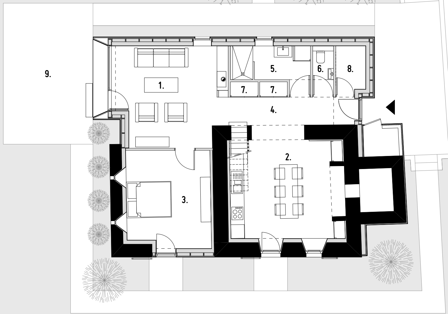
PLAN DU REZ-DE-CHAUSSÉE
