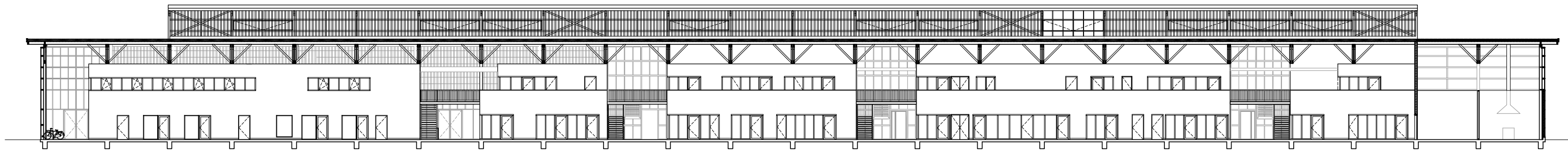
Coupe longitudinale sur bâtiment Centre-voie
