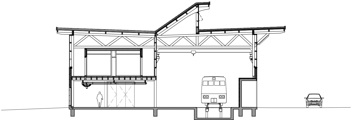
Coupe transversale sur bât.CREM
