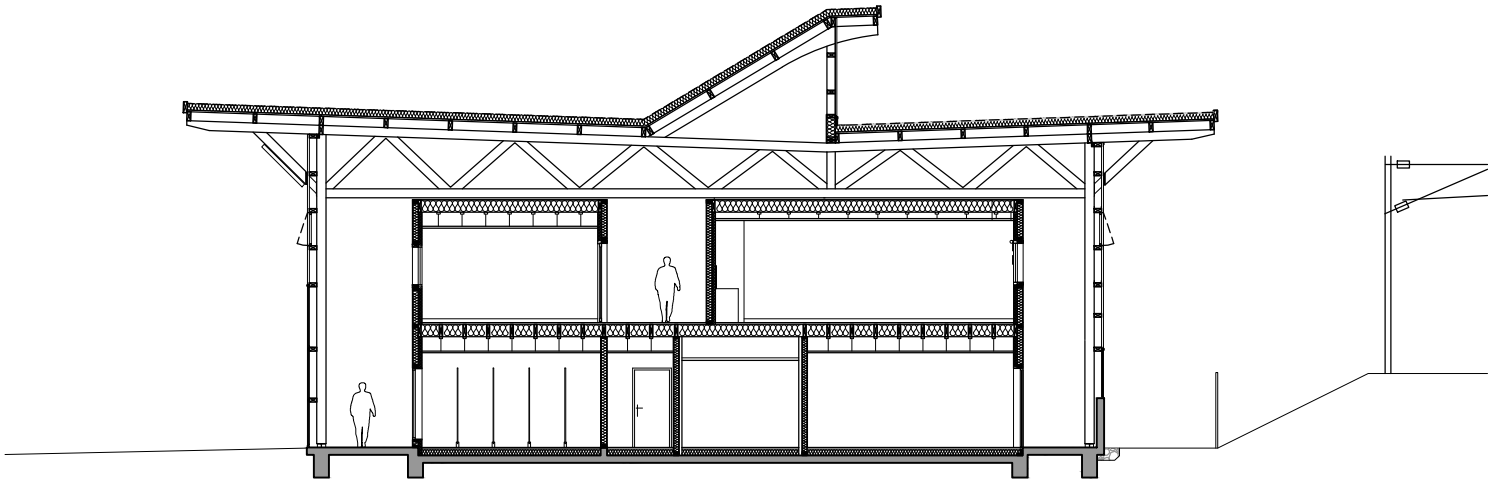
Coupe transversale sur bât.Centre-voie
