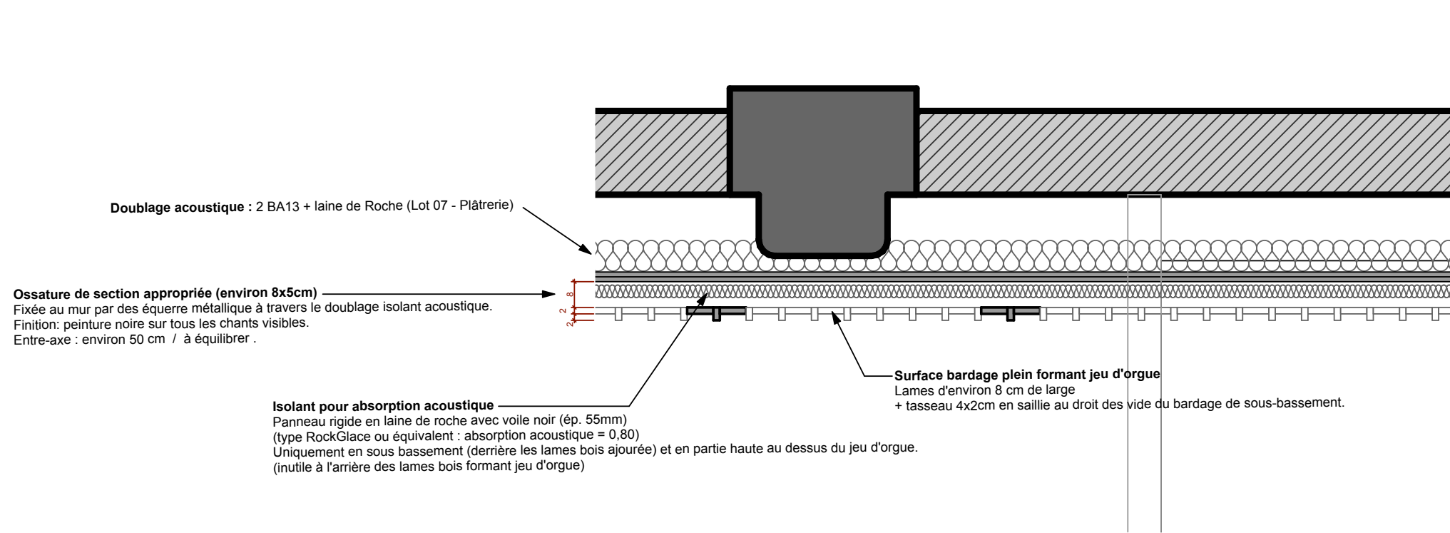
Plan Niveau 1
