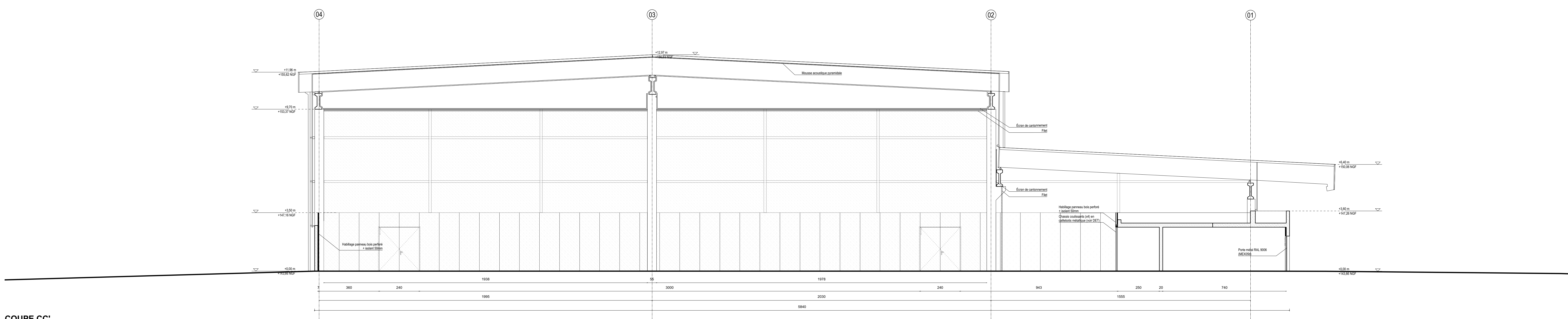
COUPE CC'
