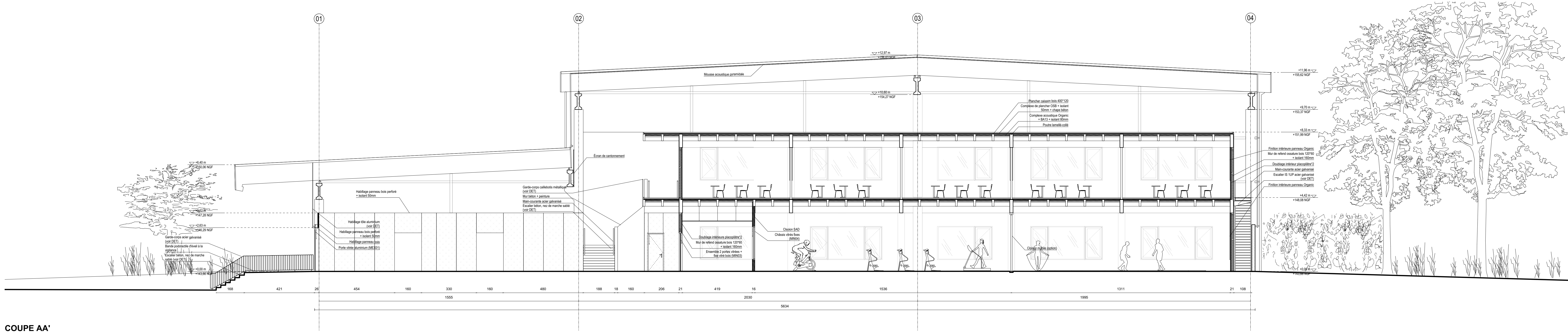
COUPE AA'
