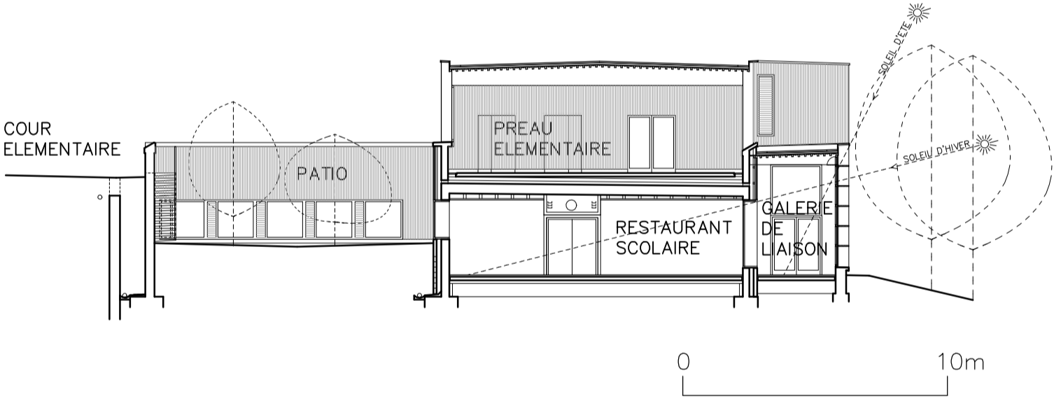
COUPE TRANSVERSALE ECHELLE: 1/200 EQUIPEMENTS SCOLAIRES A PRINGY
