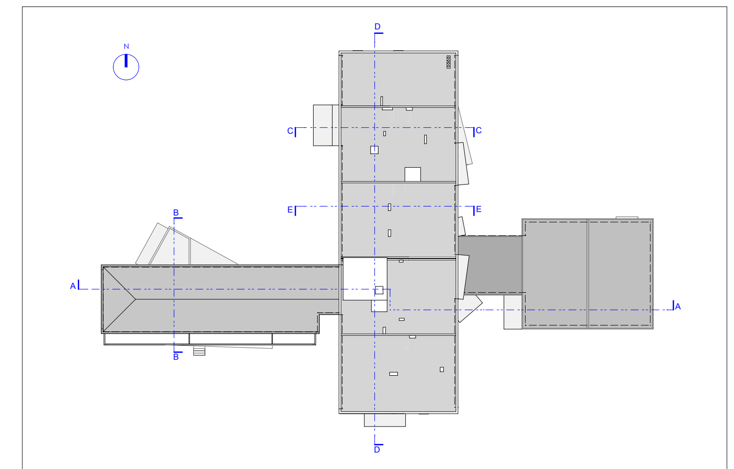
Plan de réperage - 1/500
