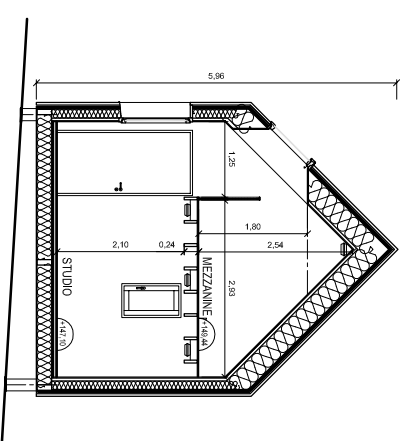
COUPE TRANSVERSALE STUDIO
