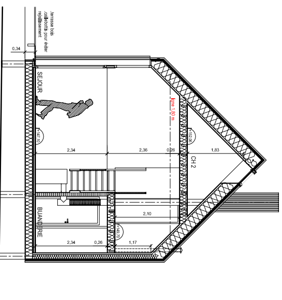
COUPE TRANSVERSALE MAISON
