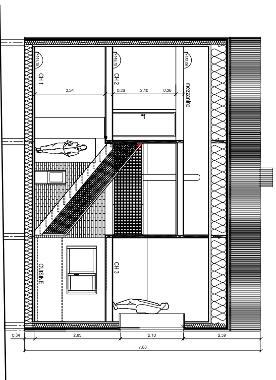
COUPE LONGITUDINALE MAISON
