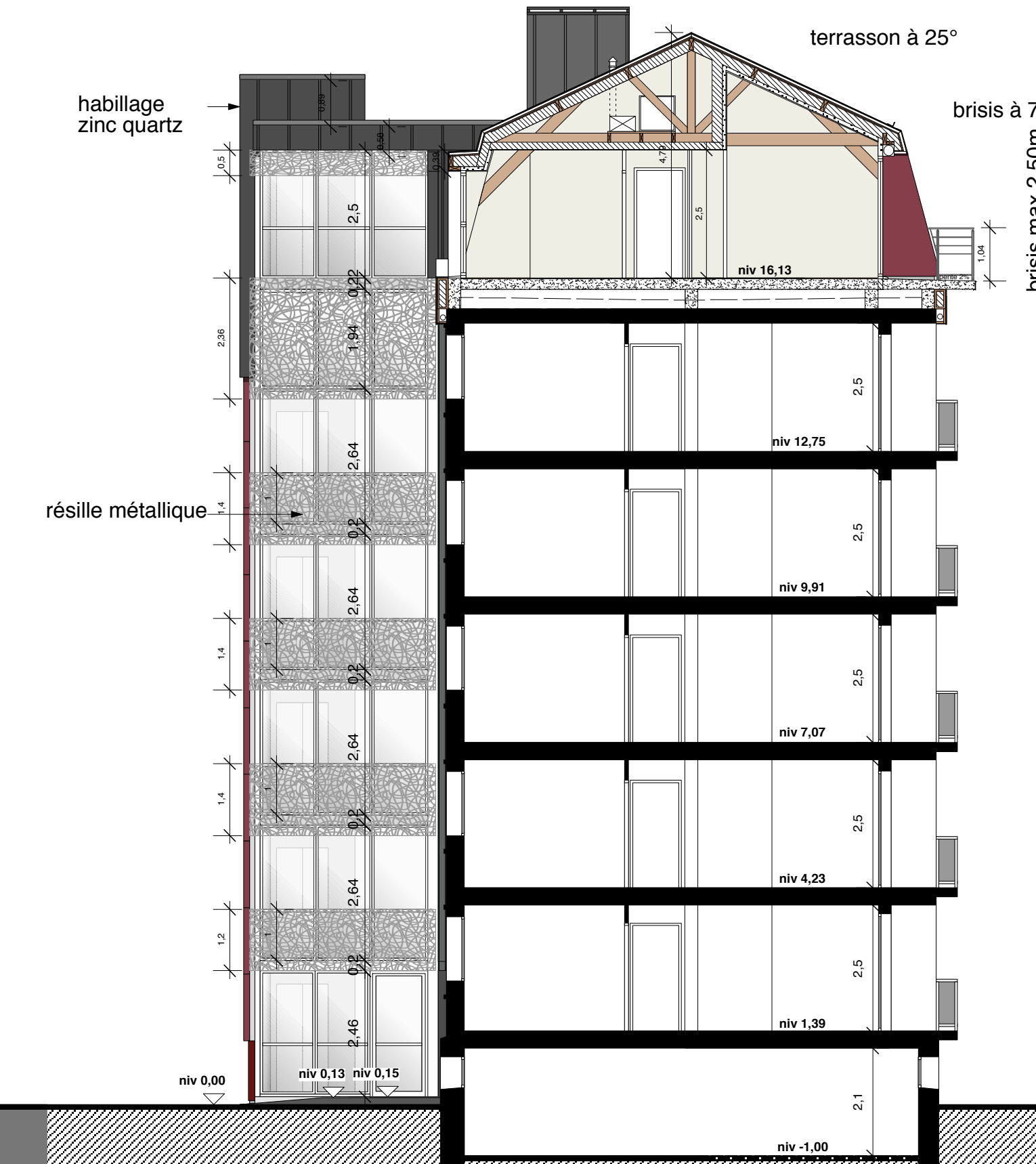
COUPE BB' - ETAT PROJETÉ
