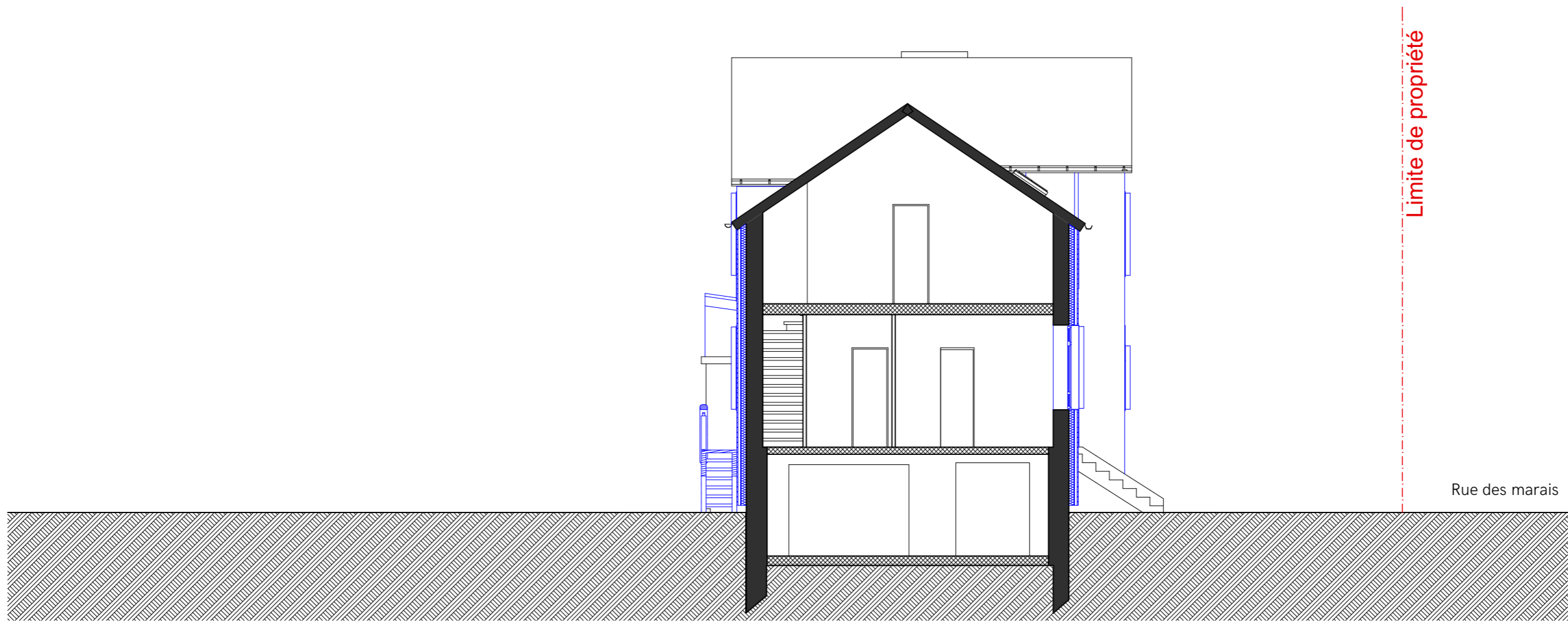
Coupe AA
