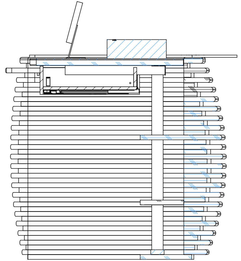
COUPE A-A
