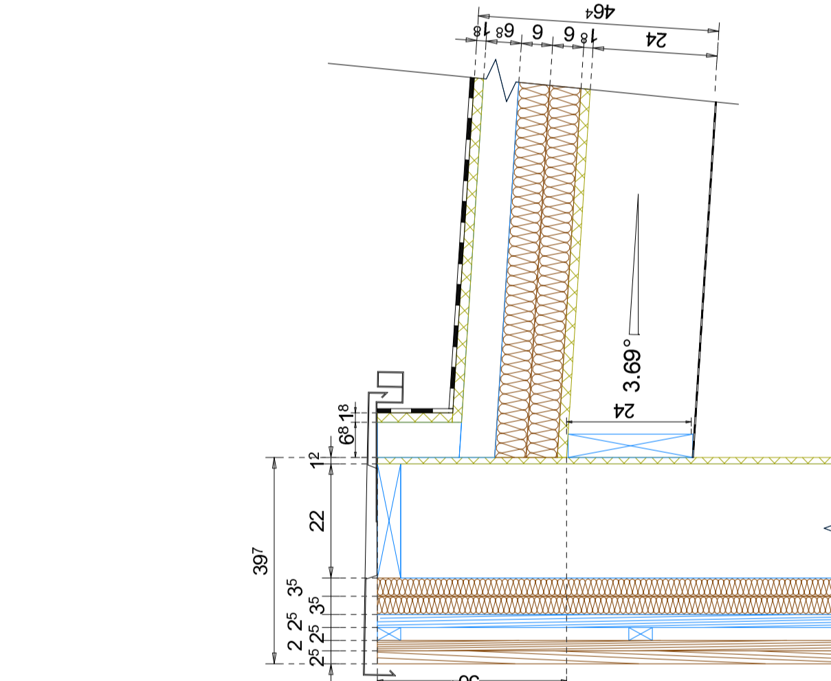
Détail B1
