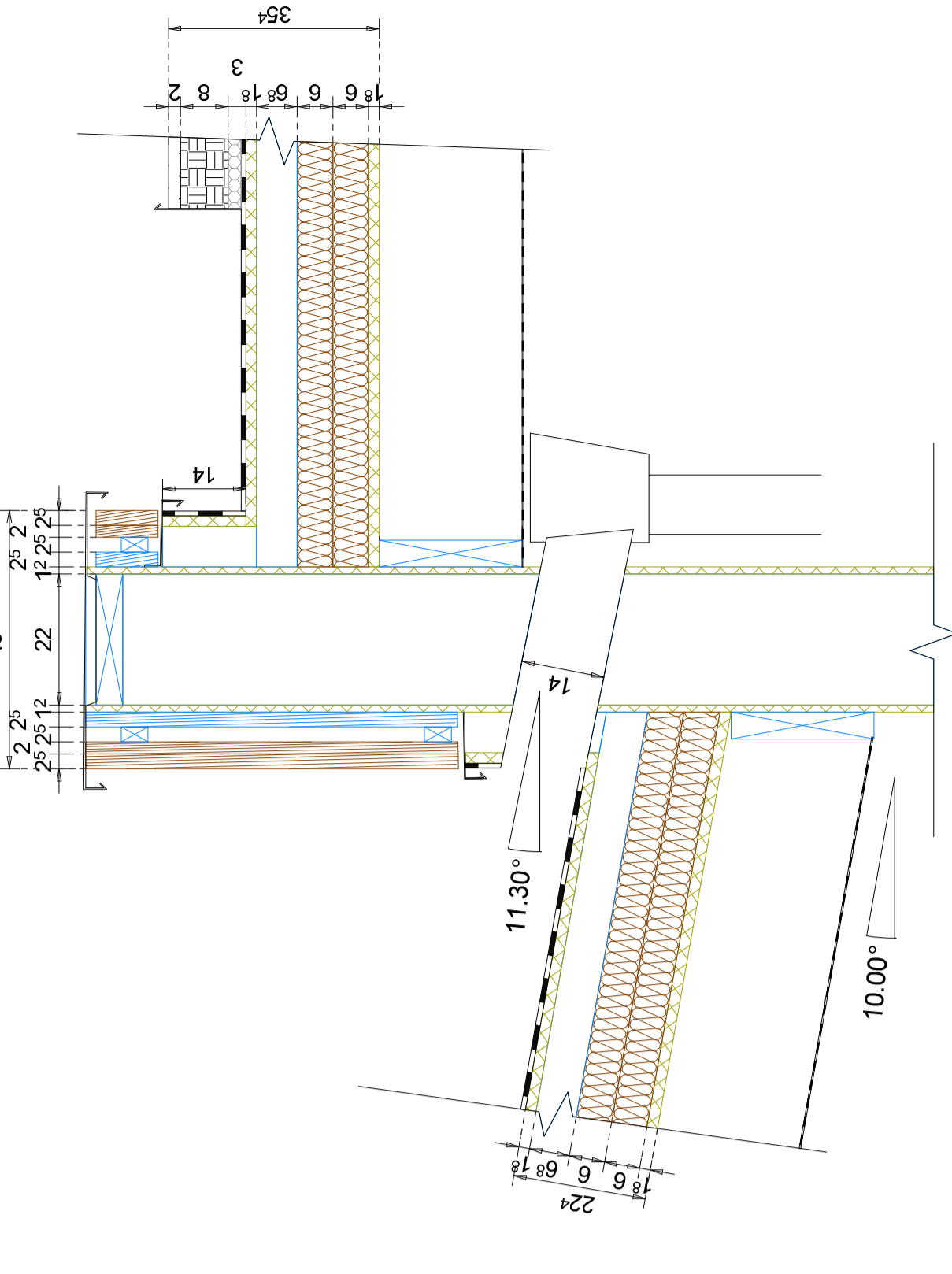
Détail A11
