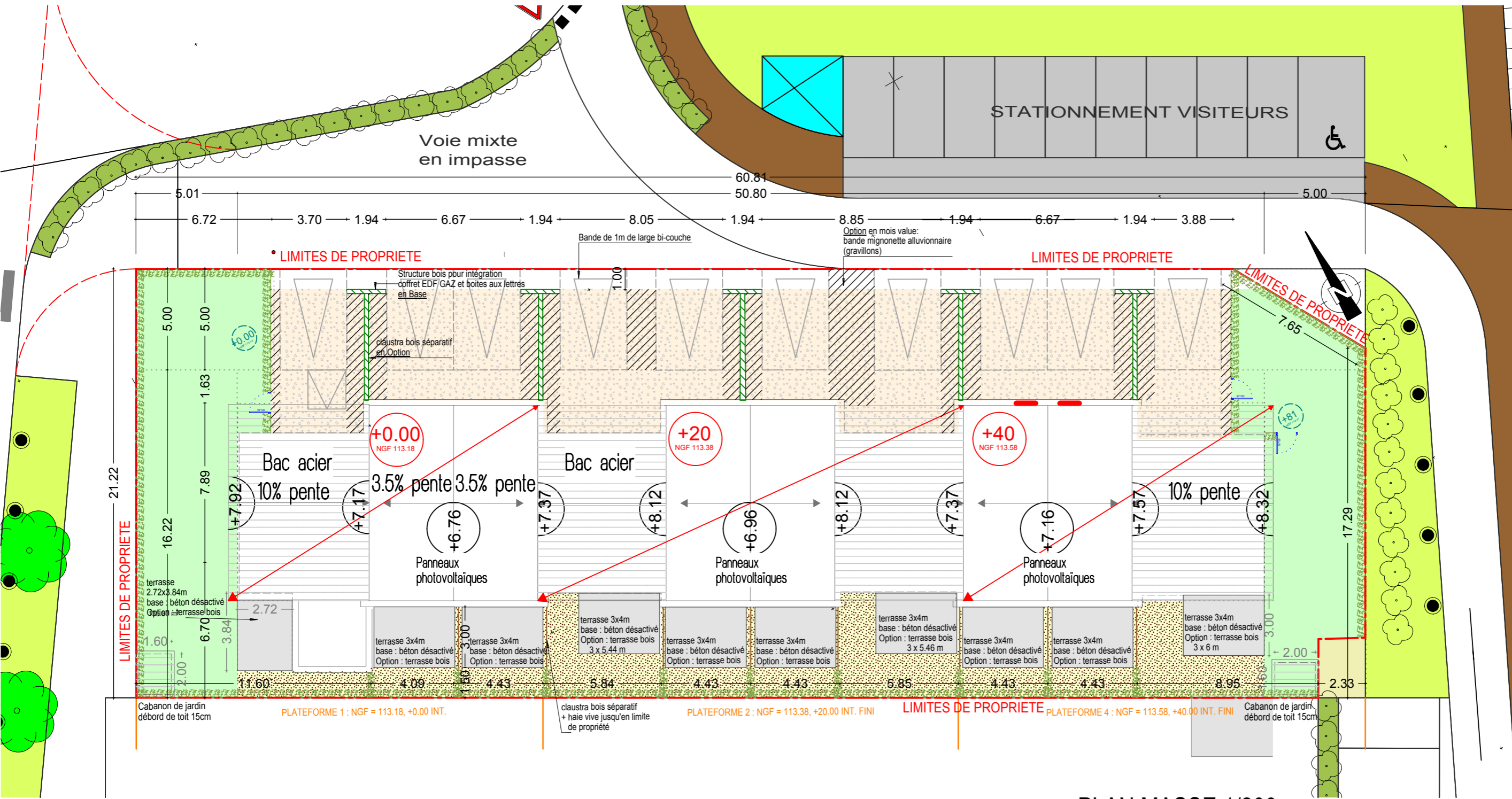
PLAN MASSE 1/200
