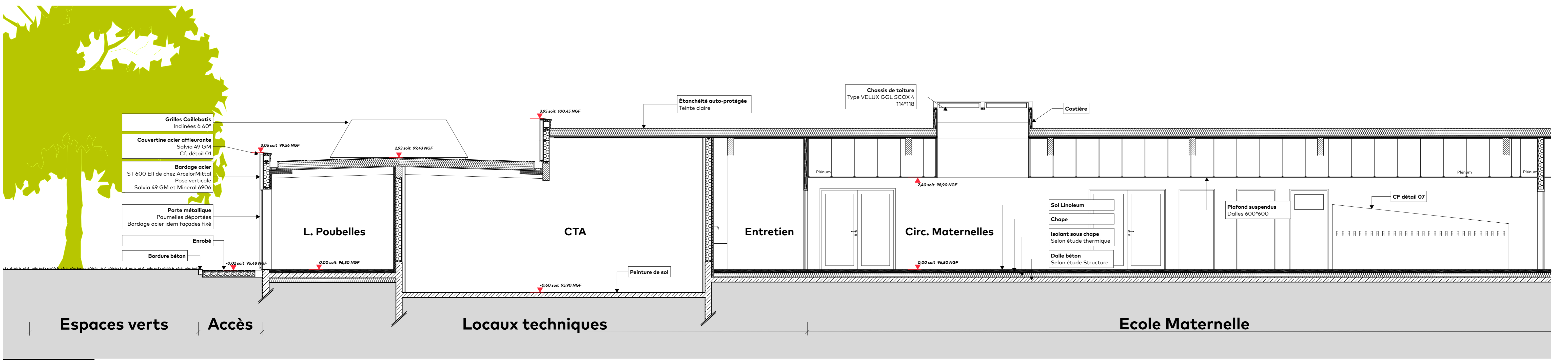
COUPE HH - Ech : 1/50
