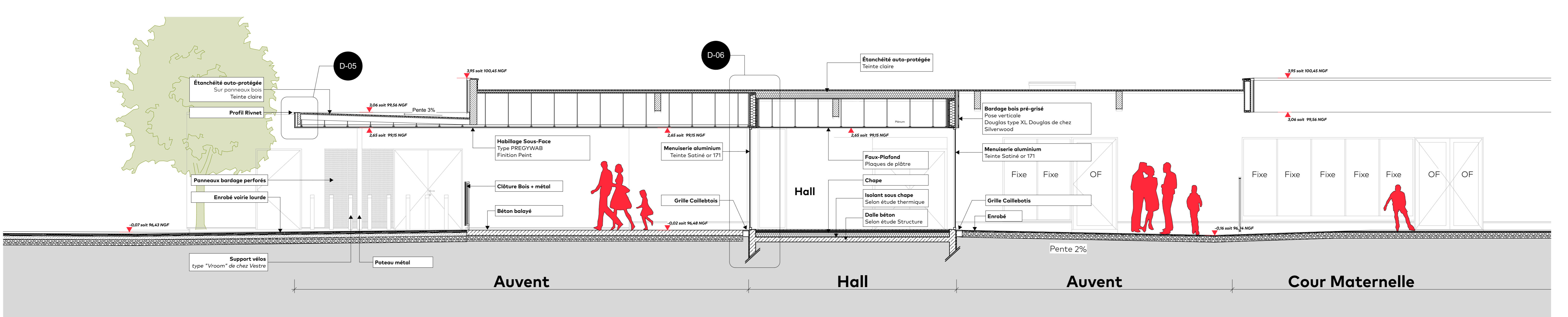
COUPE II - Ech : 1/50
