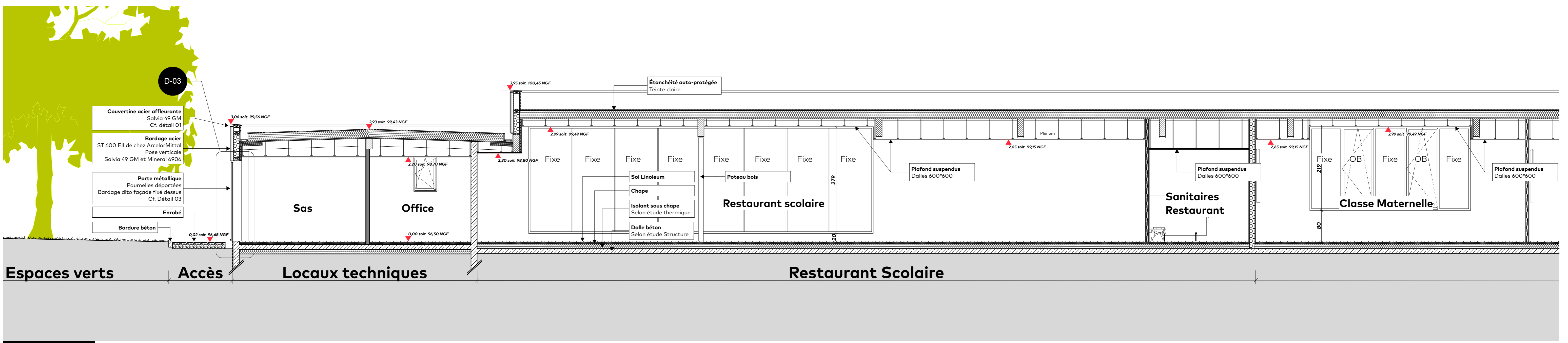
COUPE GG - Ech : 1/50
