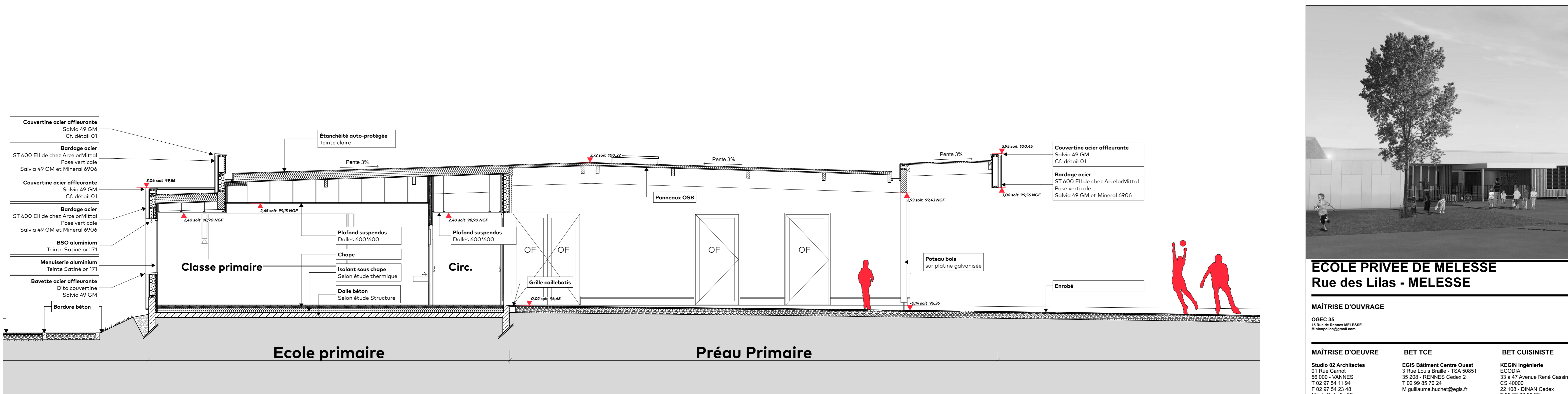
COUPE KK - Ech : 1/50
