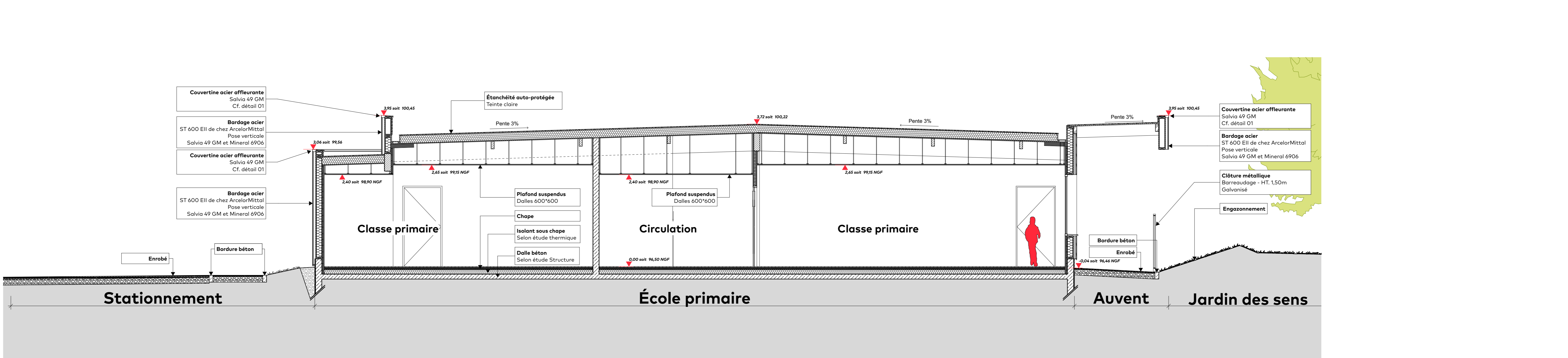
COUPE JJ - Ech : 1/50
