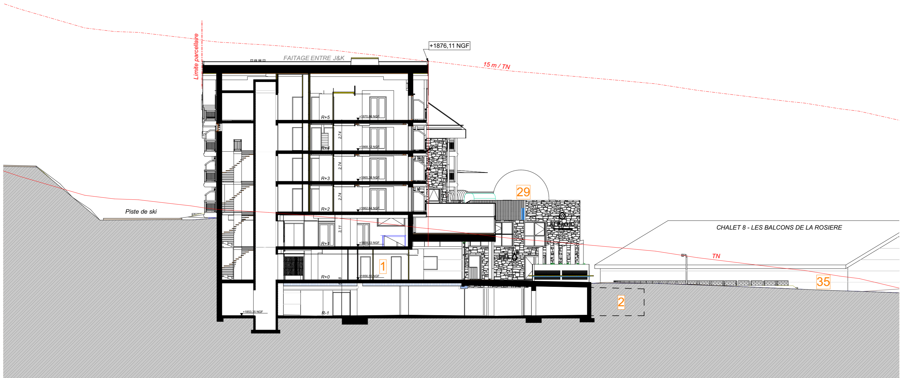
COUPE PAYSAGERE
