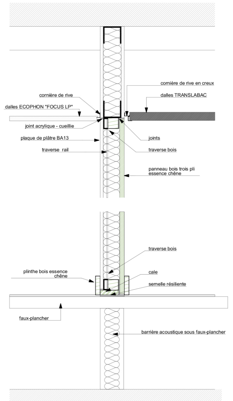
CLOISON BOIS/PLÂTRE SOUS IMPOSTE
