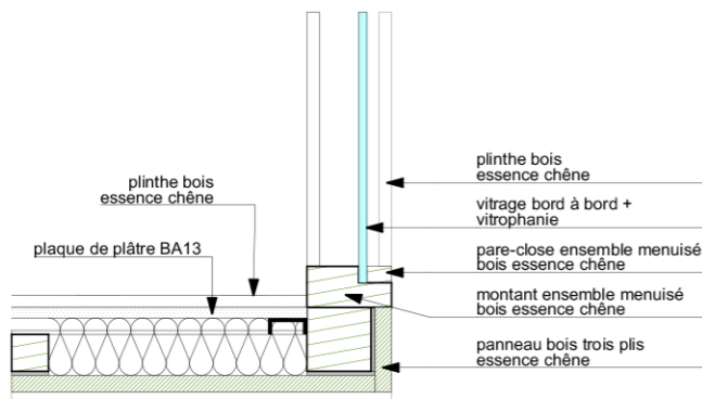
CLOISON VITRÉE SOUS IMPOSTE
