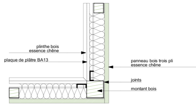
CLOISON BOIS/BOIS SOUS IMPOSTE
