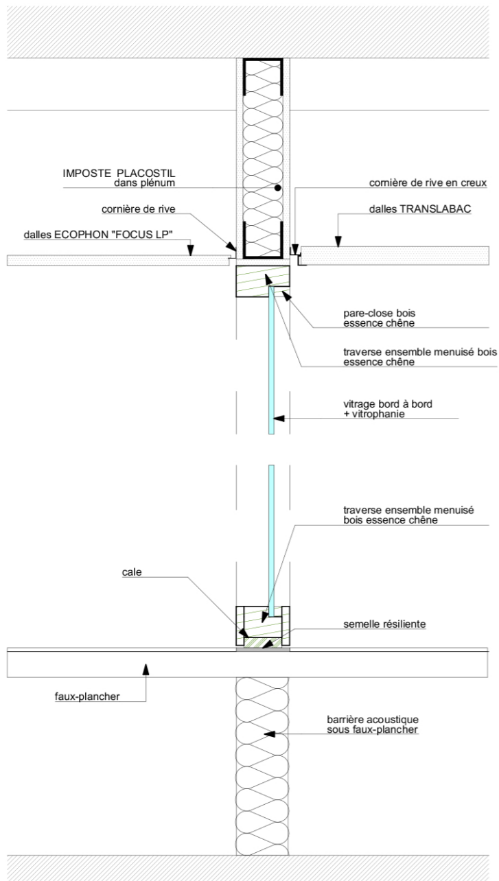
CLOISON VITRÉE SOUS IMPOSTE
