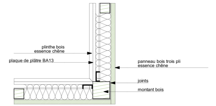
CLOISON BOIS/PLÂTRE SOUS IMPOSTE
