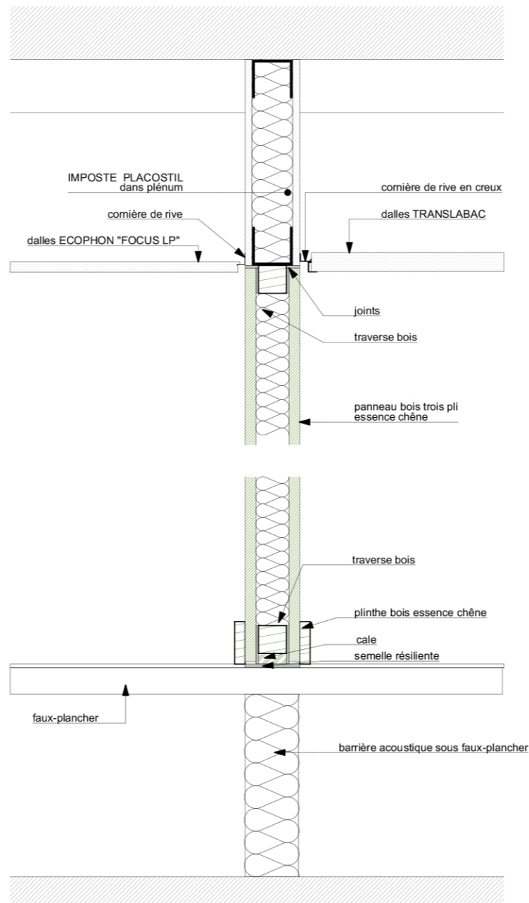
CLOISON BOIS/BOIS SOUS IMPOSTE
