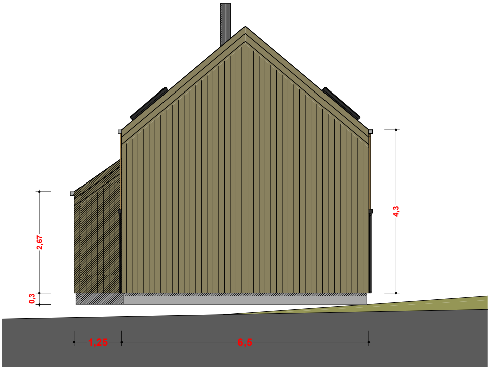
FACADE NORD OUEST
