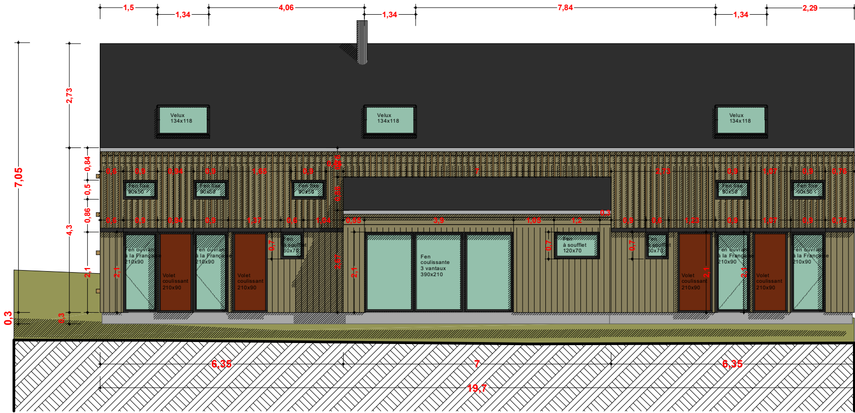
FACADE NORD EST
