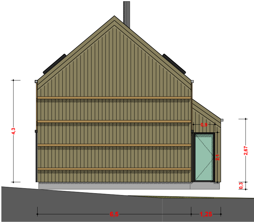
FACADE SUD EST
