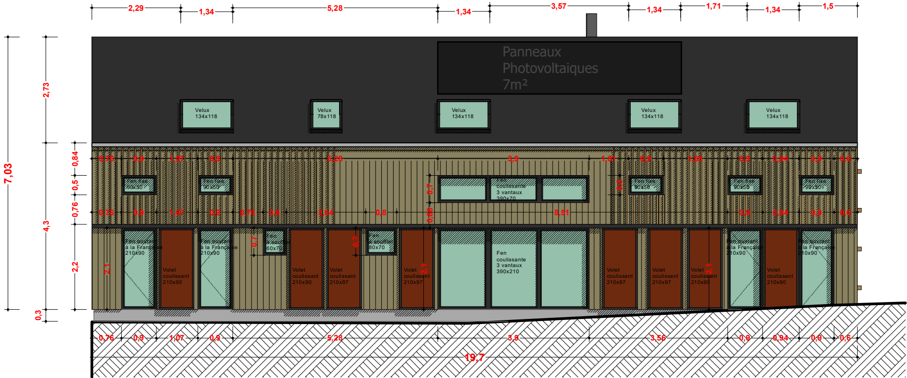
FACADE SUD OUEST
