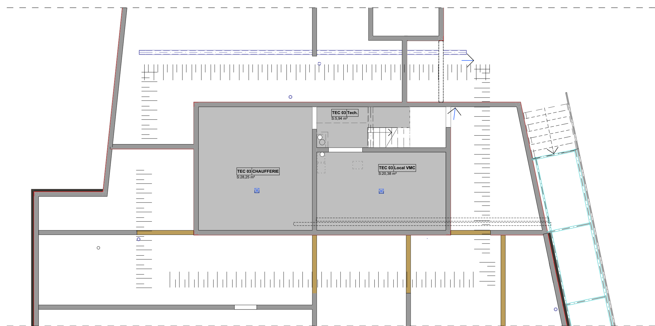
Plan de niveau Sous-sol / vide technique, échelle 1/100ème
