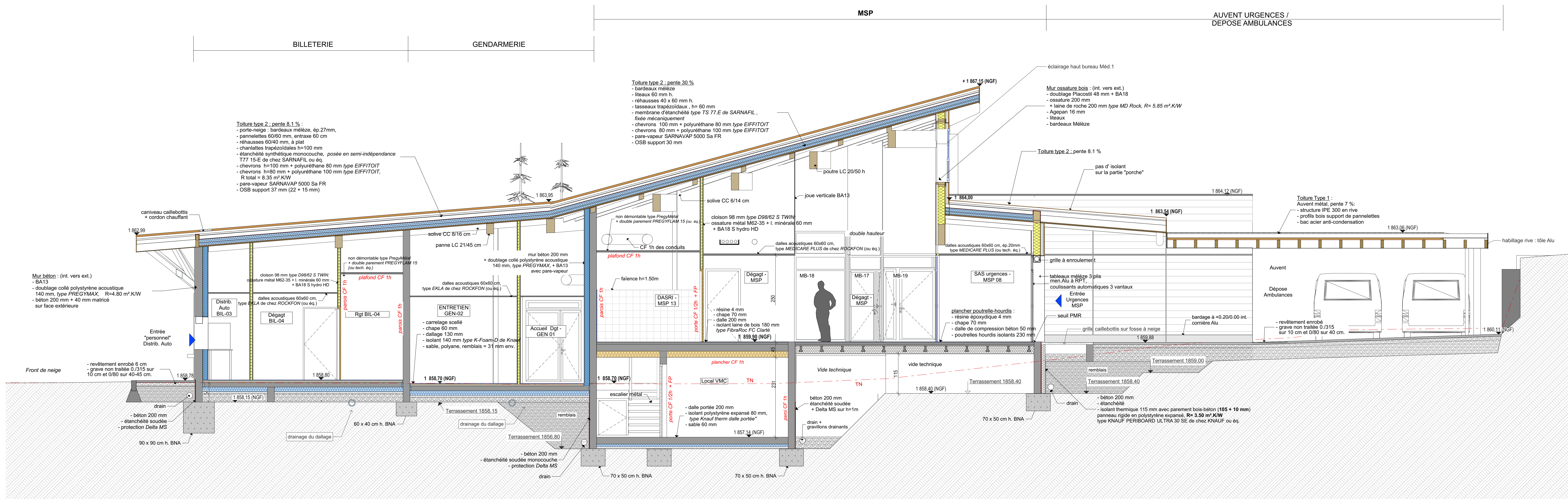
Coupe longitudinale L1 - sur Auvent Urgences
