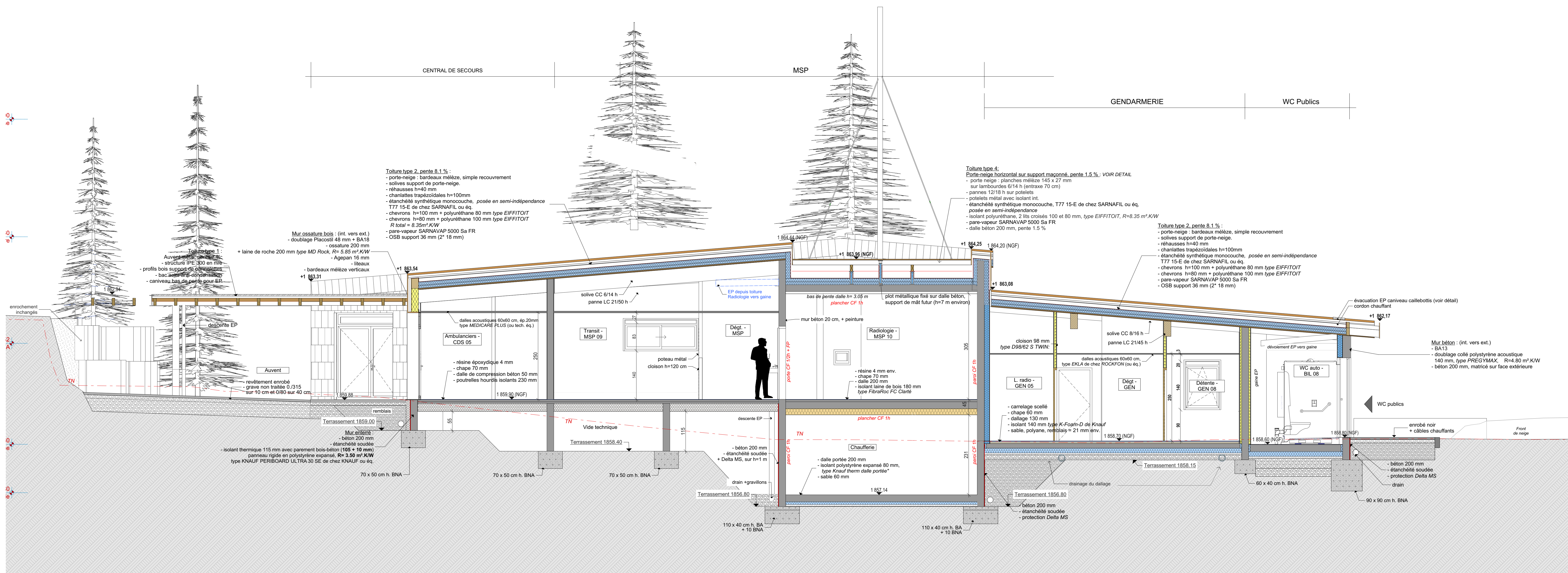
Coupe longitudinale L2 - sur Radiologie et Chauffage
