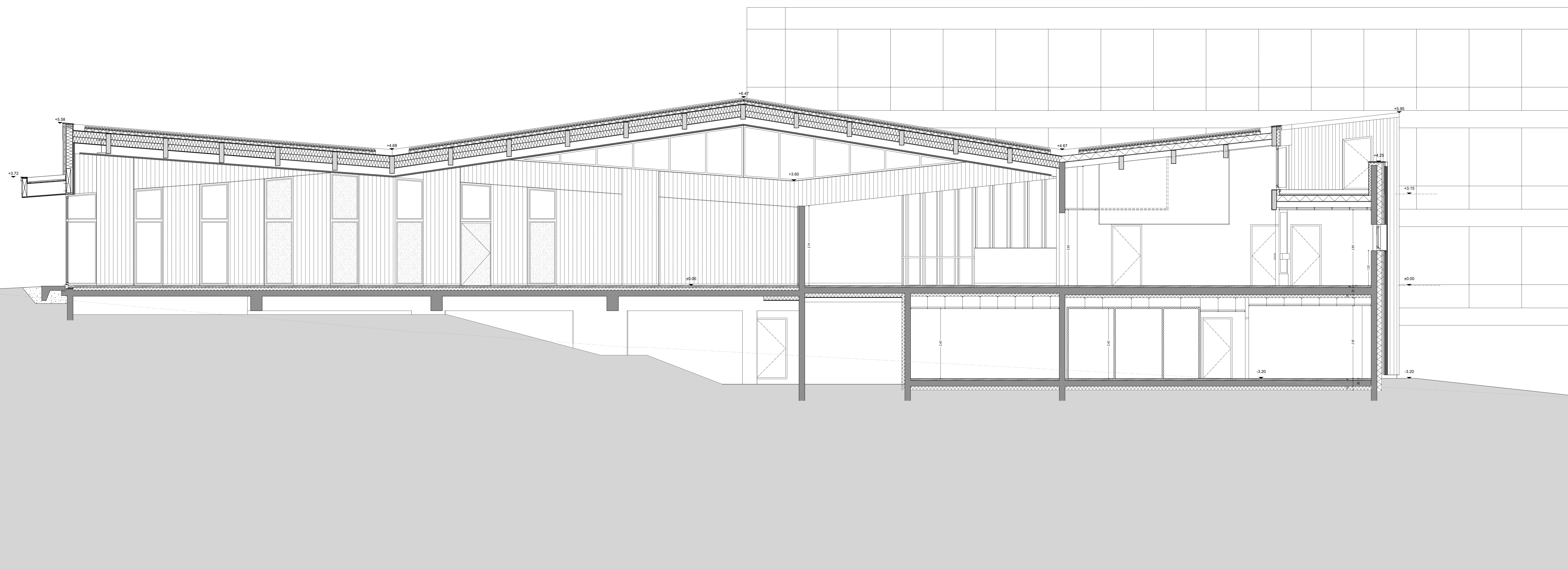
COUPE LONGITUDINALE
