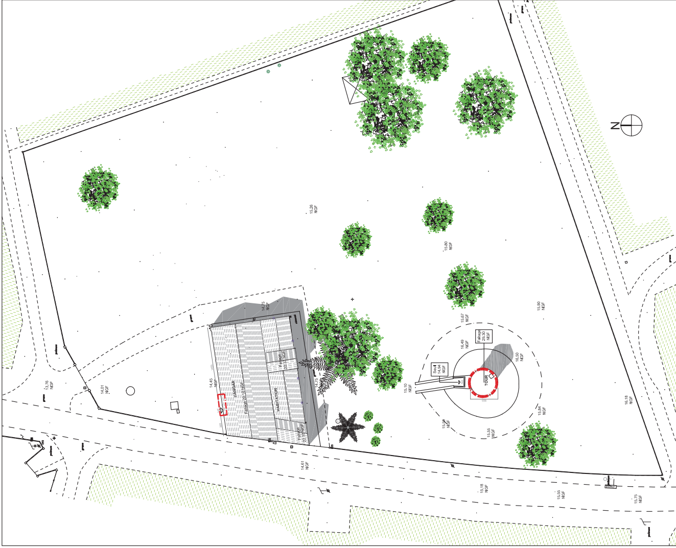
PLAN éch. 200ème - source Michel MARTIN Geometre-Expert
