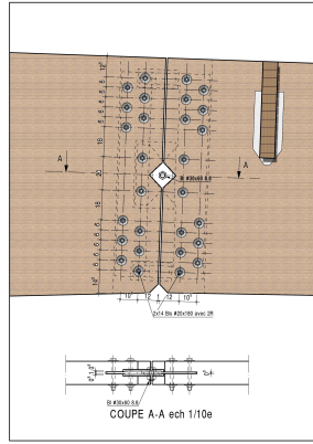
DETAIL 5 ech 1/10e
