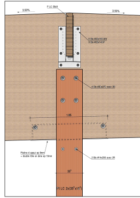
DETAIL 3 ech 1/10e
