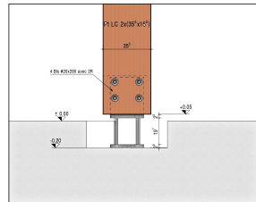
DETAIL 4 ech 1/10e
