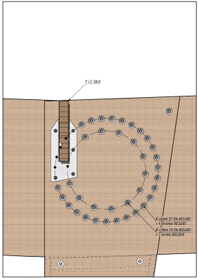
DETAIL 1 ech 1/10e
