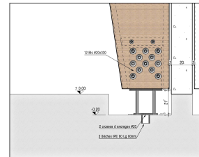
DETAIL 7 ech 1/10e
