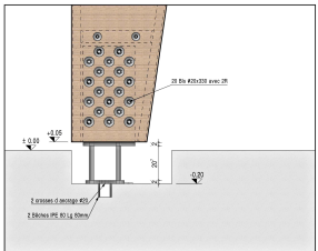
DETAIL 2 ech 1/10e
