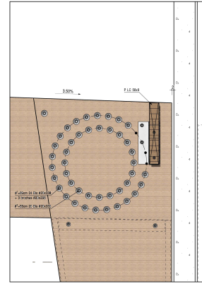
DETAIL 6 ech 1/10e
