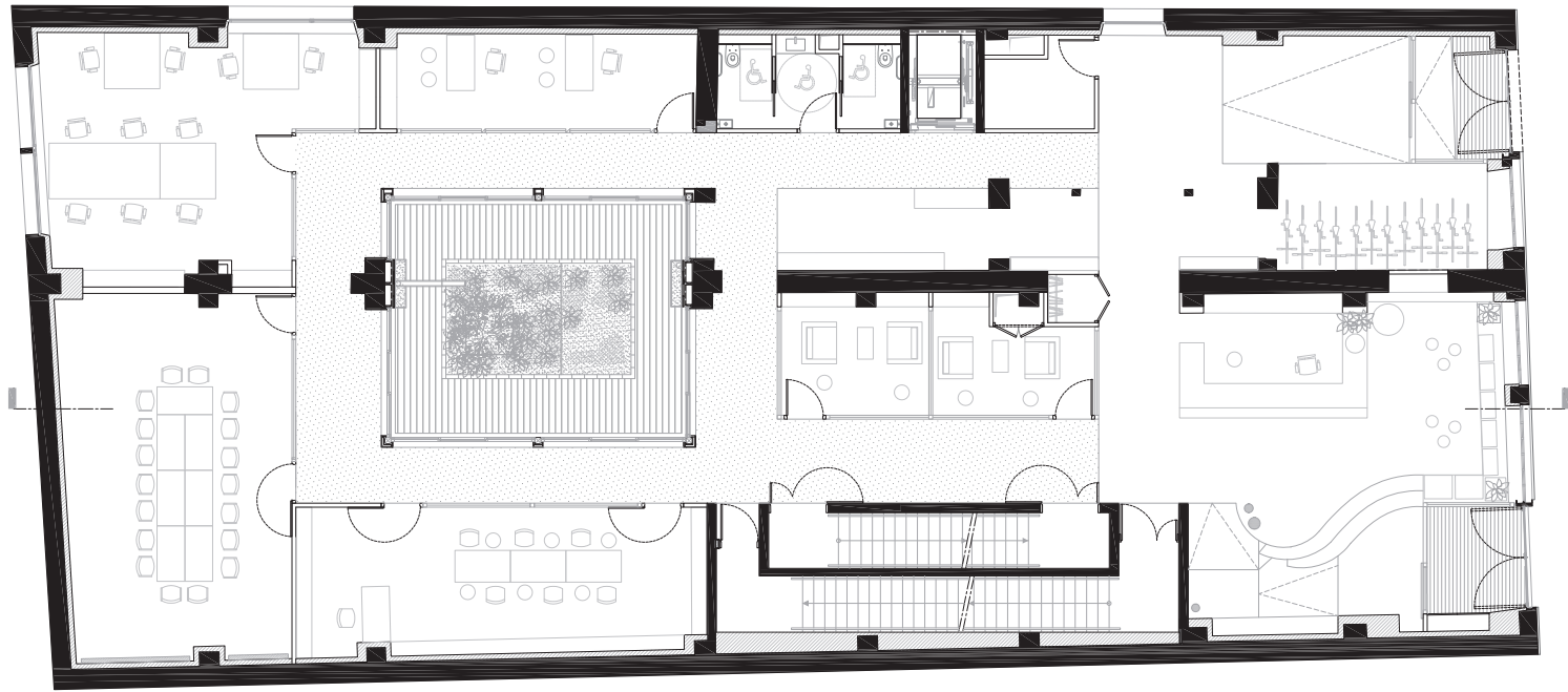
RDC 0 1 2 3 4 5m
