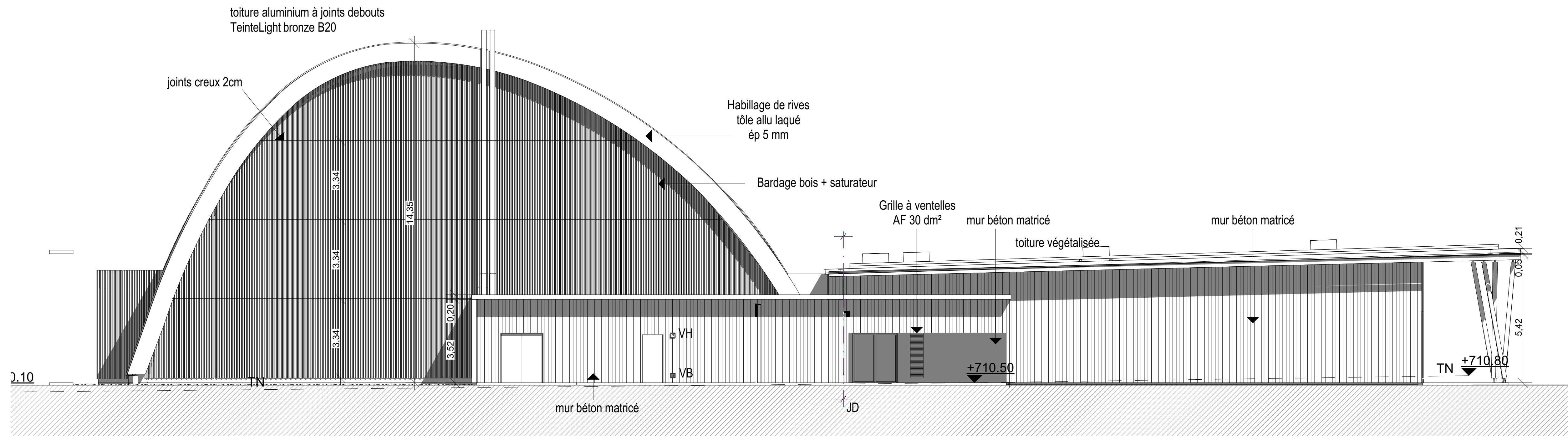
FACADE OUEST - Echelle 1 : 100
