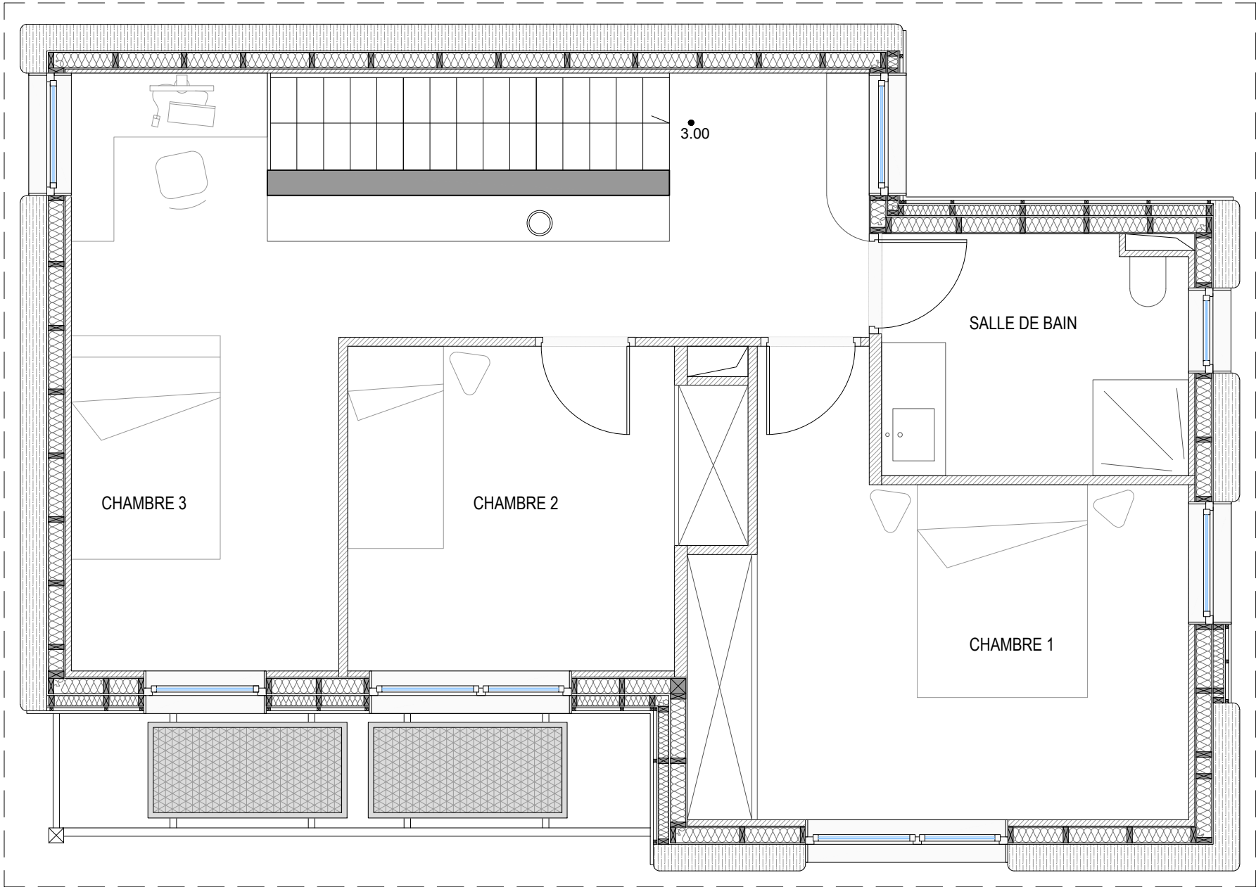
PLAN DE L'ETAGE
