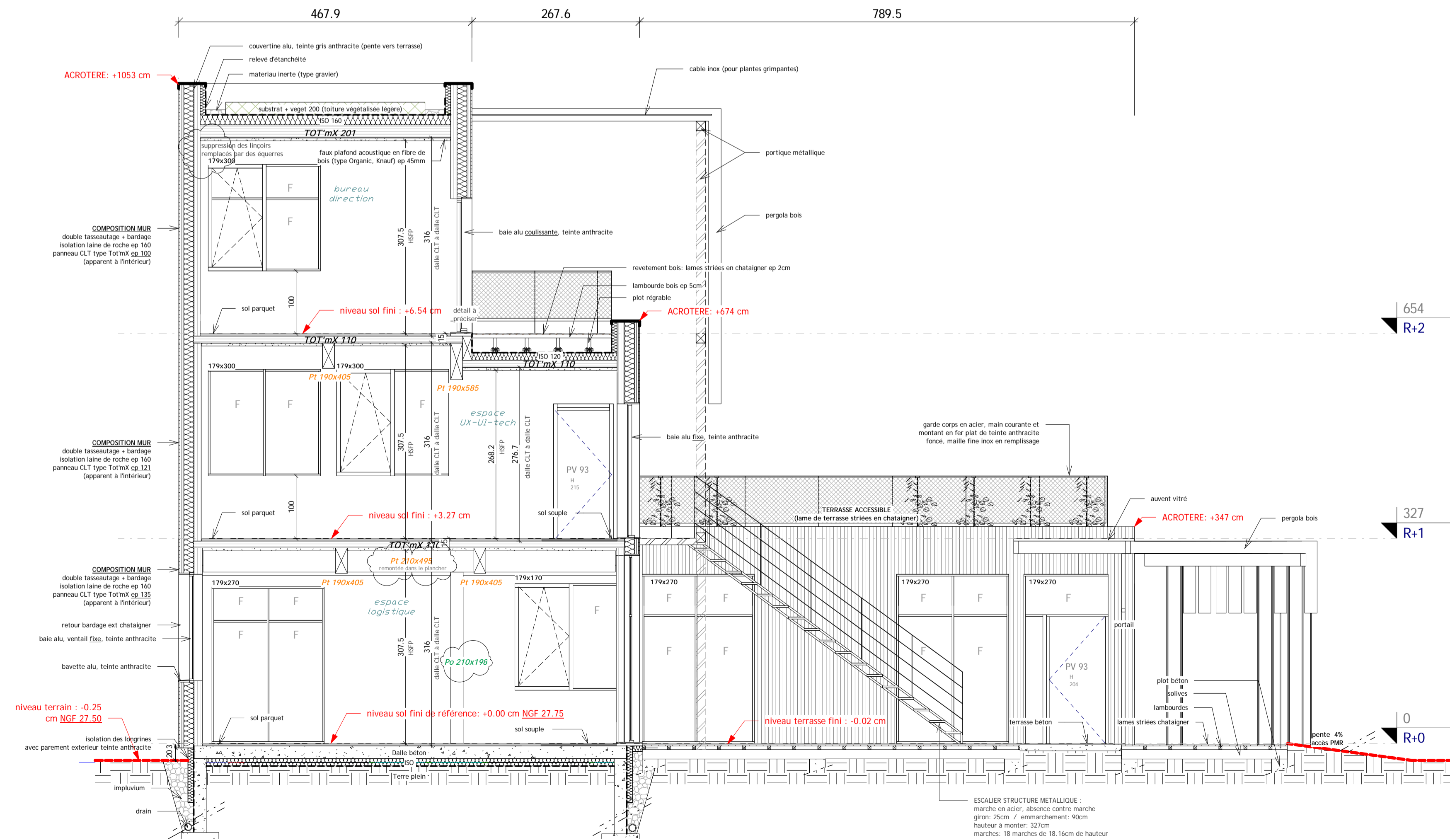
1 Coupe 1 - E/O Ech : 1 : 50
