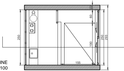
PLAN RDC 1/100
